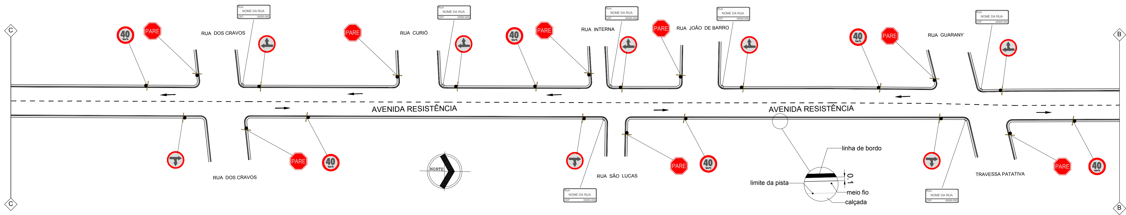
PLANTA DE SINALIZAÇÃO escala: 1/500
