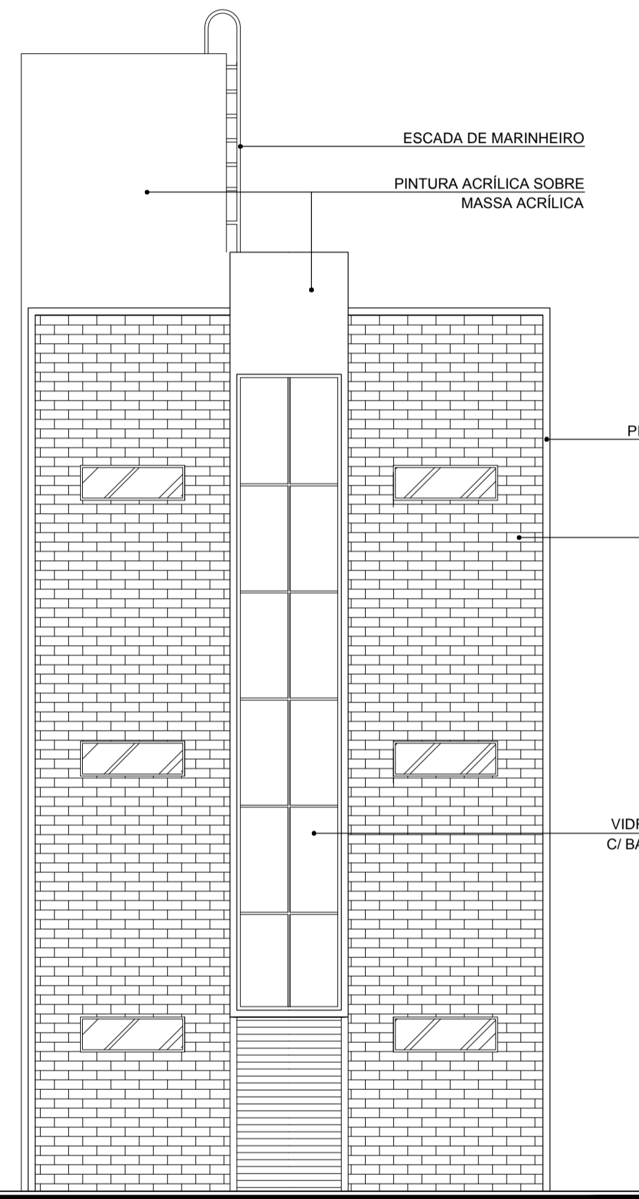
FACHADA 03 ESC.: 1/75
