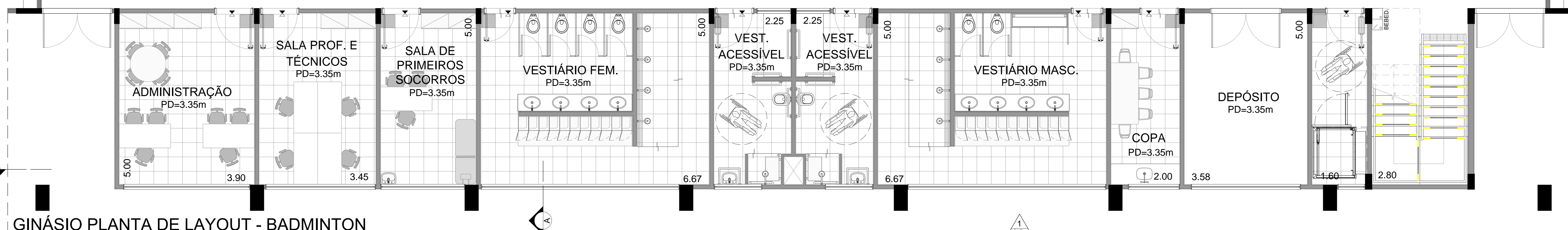
GINÁSIO PLANTA DE LAYOUT - BADMINTON ESC. 1:50
