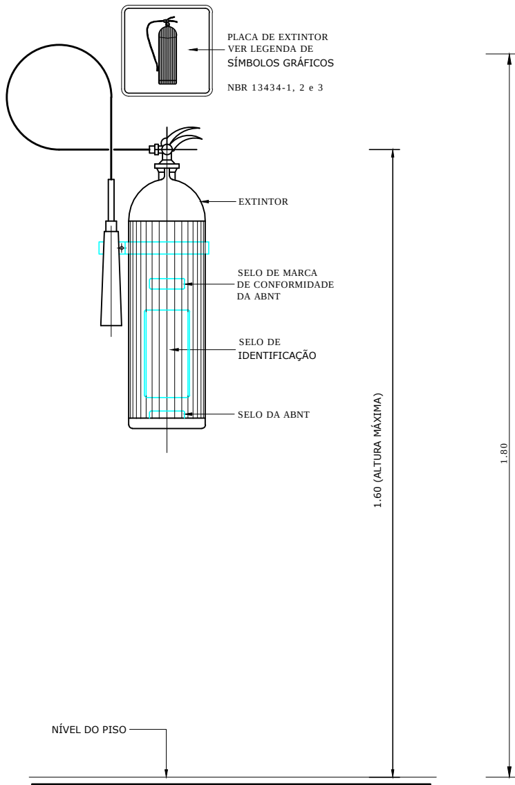
DETALHE 02 - EXTINTOR SEM ESCALA
