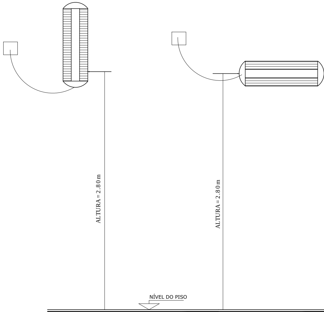
DETALHE 01- ILUMINAÇÃO DE EMERGÊNCIA SEM ESCALA
