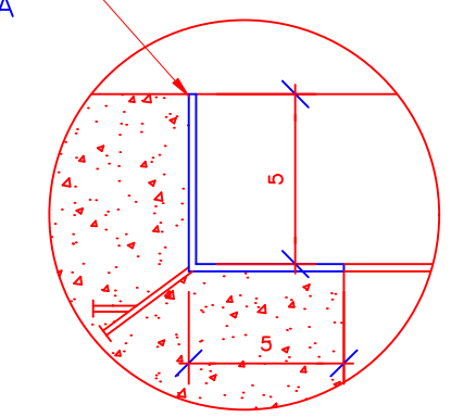
TAMPA DE CONCRETO DETALHE 02 Esc.: sem escala
