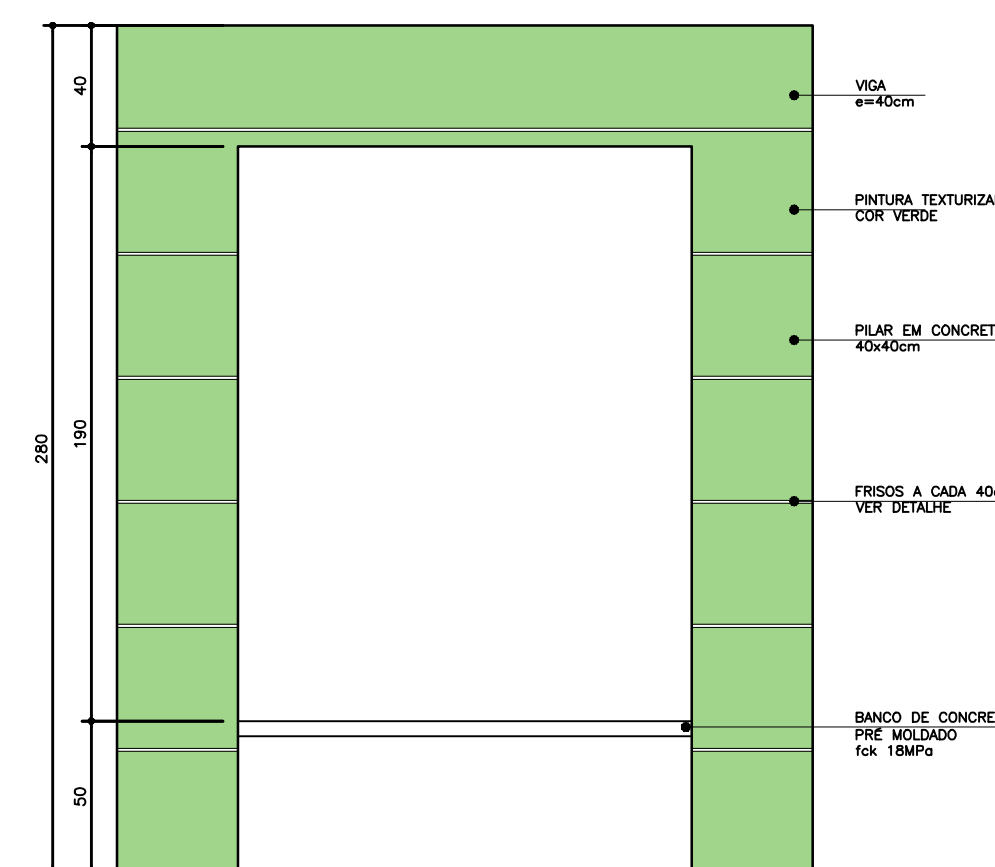
Elevação 01
