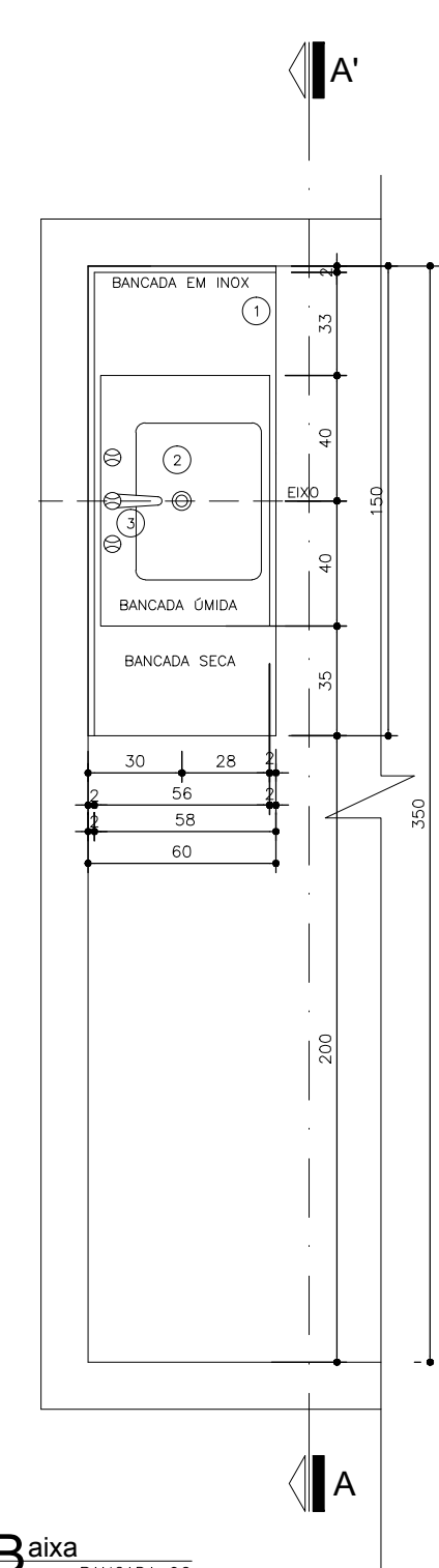
Planta Baixa
