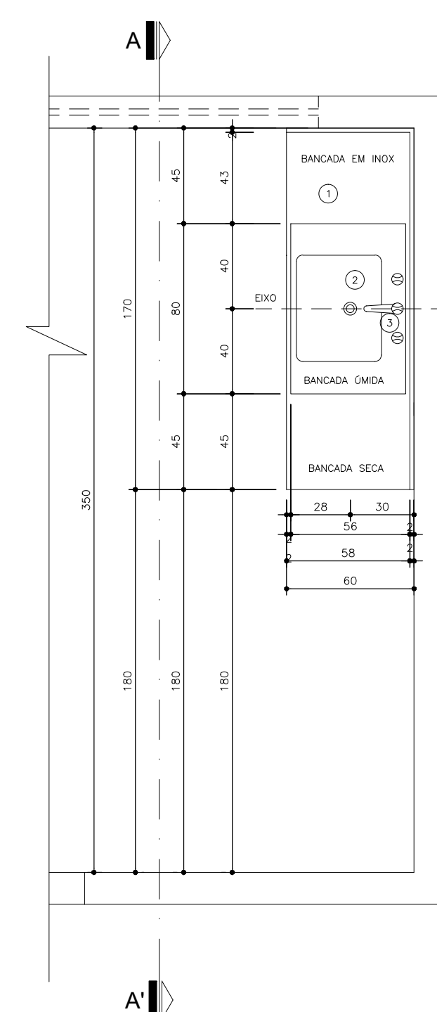
Planta Baixa
