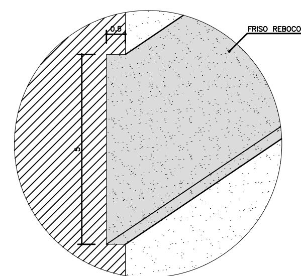
Detalhe Friso
