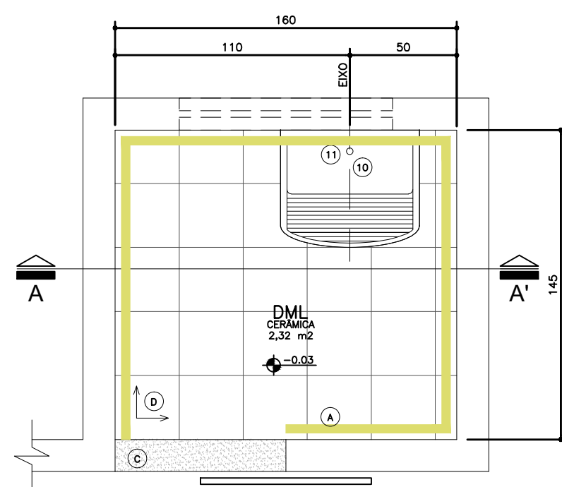
01 Planta Baixa Amb. 01 - DML Esc.: 1:25
