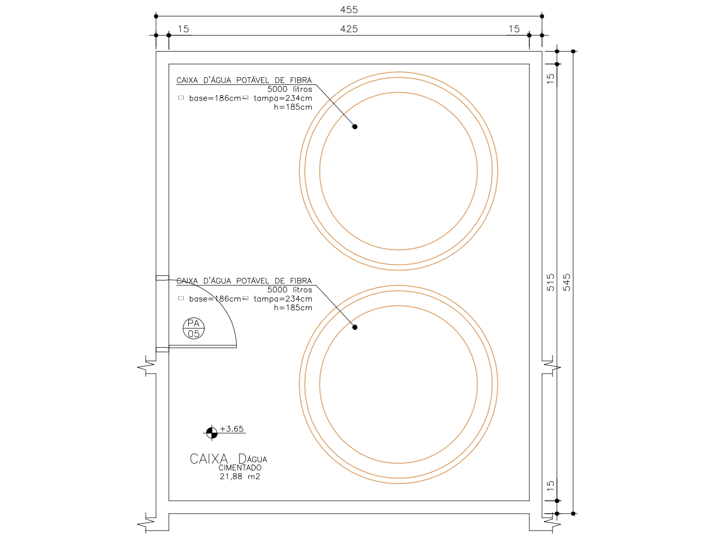
Planta Baixa Caixa D'água
