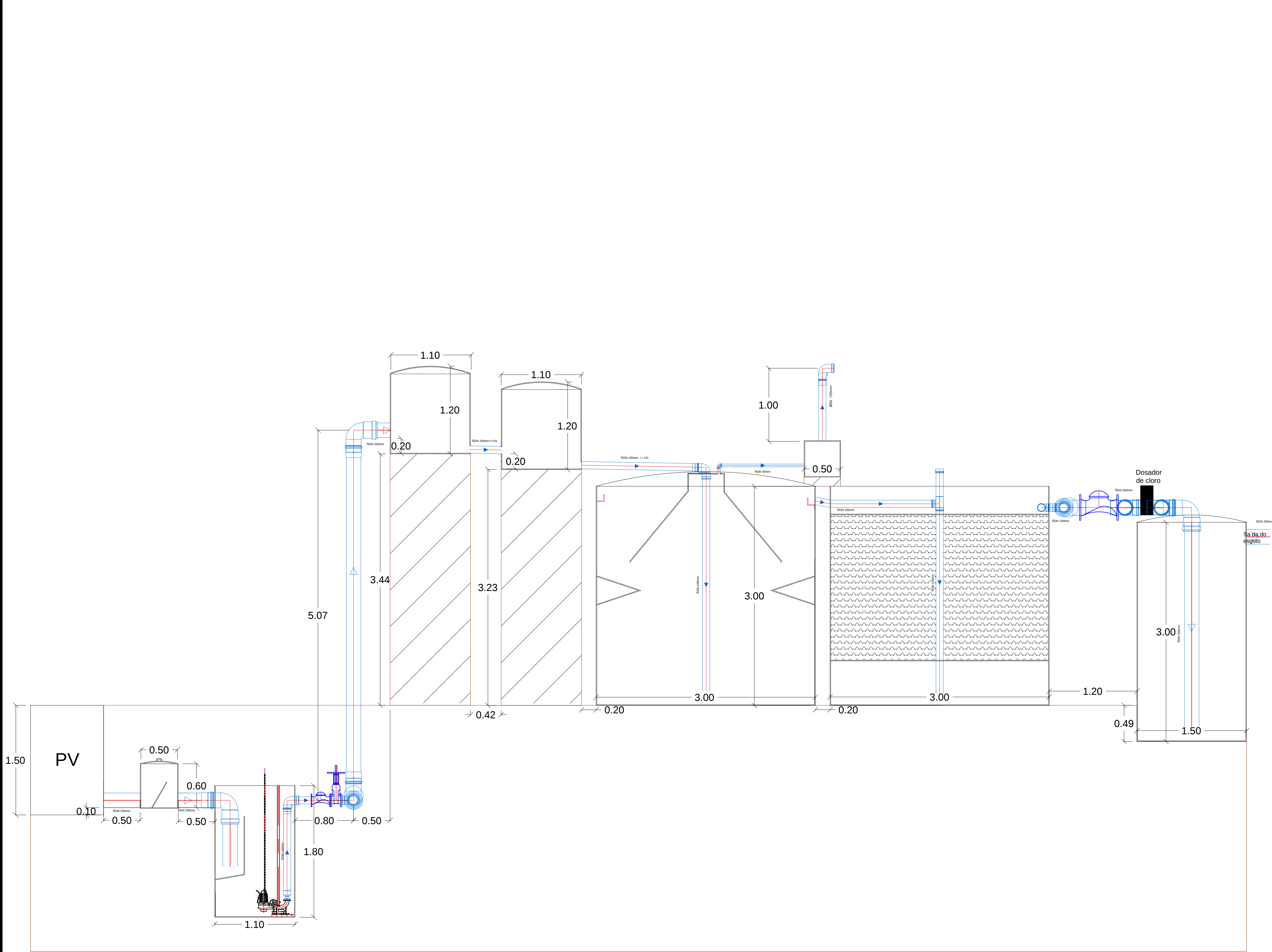
CORTE INSTALAÇÃO ETE MAIOR Esc. 1/30
