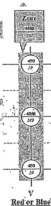
FIGURA 3-- REQUISITOS FOTOMÉTRICOS CLASSE 1 - VERMELHO Potência Óptica (Cd-segundos/Minuto) visualizado em Bold (valor superior) Pico de Intensidade Luminosa (Candela) visualizado em Itálico (valor inferior) Fonte: SAE J845 Revised AUG2021, Page 14 of 18.
