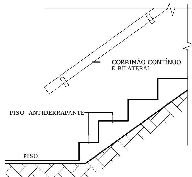
ESCADA E CORRIMÃO
