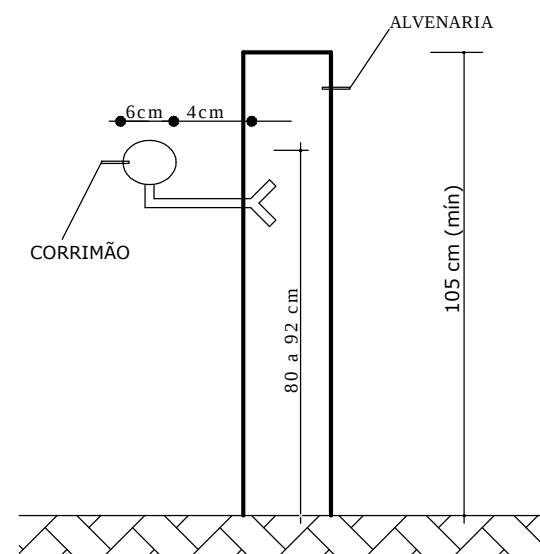
CORRIMÃO FIXADO NA PAREDE
