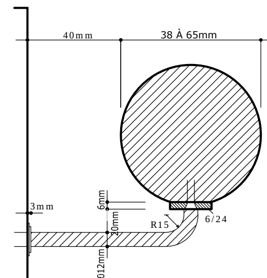
FIXAÇÃO DO CORRIMÃO
