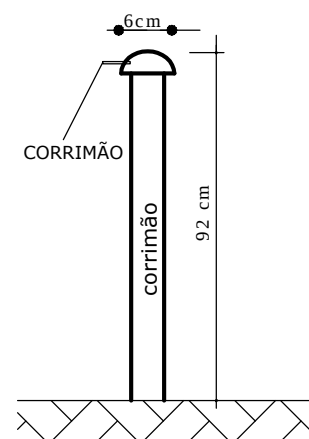
CORRIMÃO E GUARDA-CORPO
