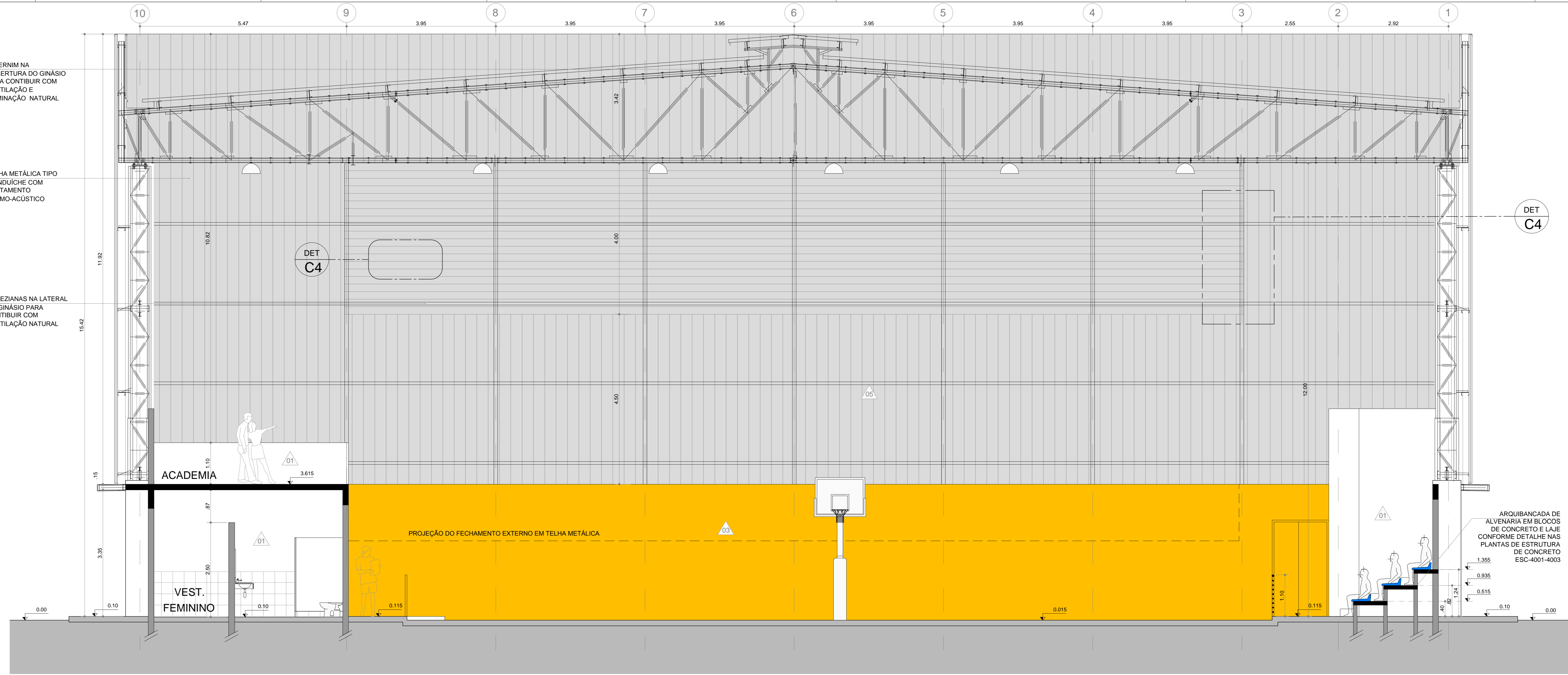
GINÁSIO - CORTE A ESC. 1:50
