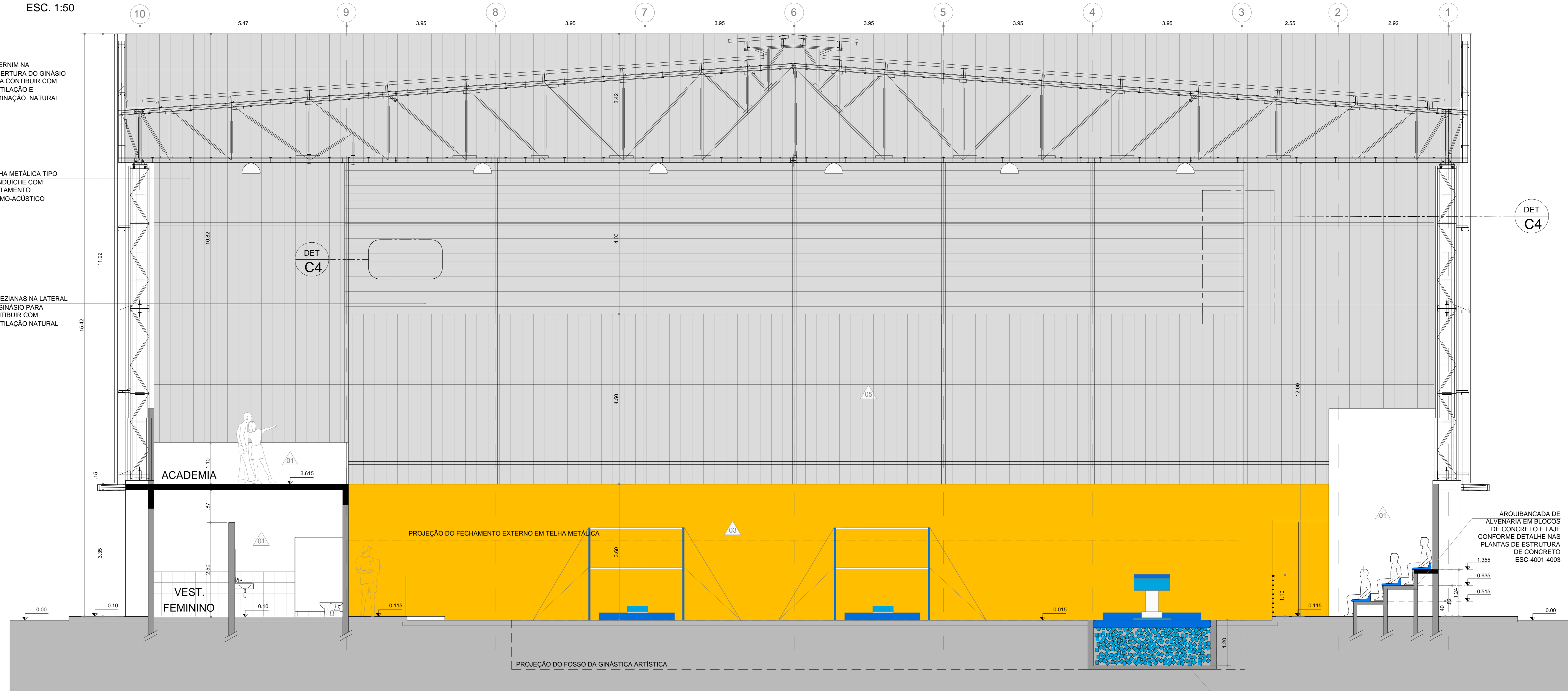
GINÁSIO - CORTE A (APENAS PARA GINÁSTICA ARTÍSTICA) ESC. 1:50
