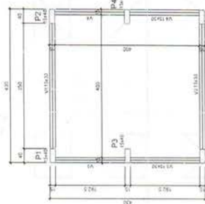
Forma do pavimento Baldrame
