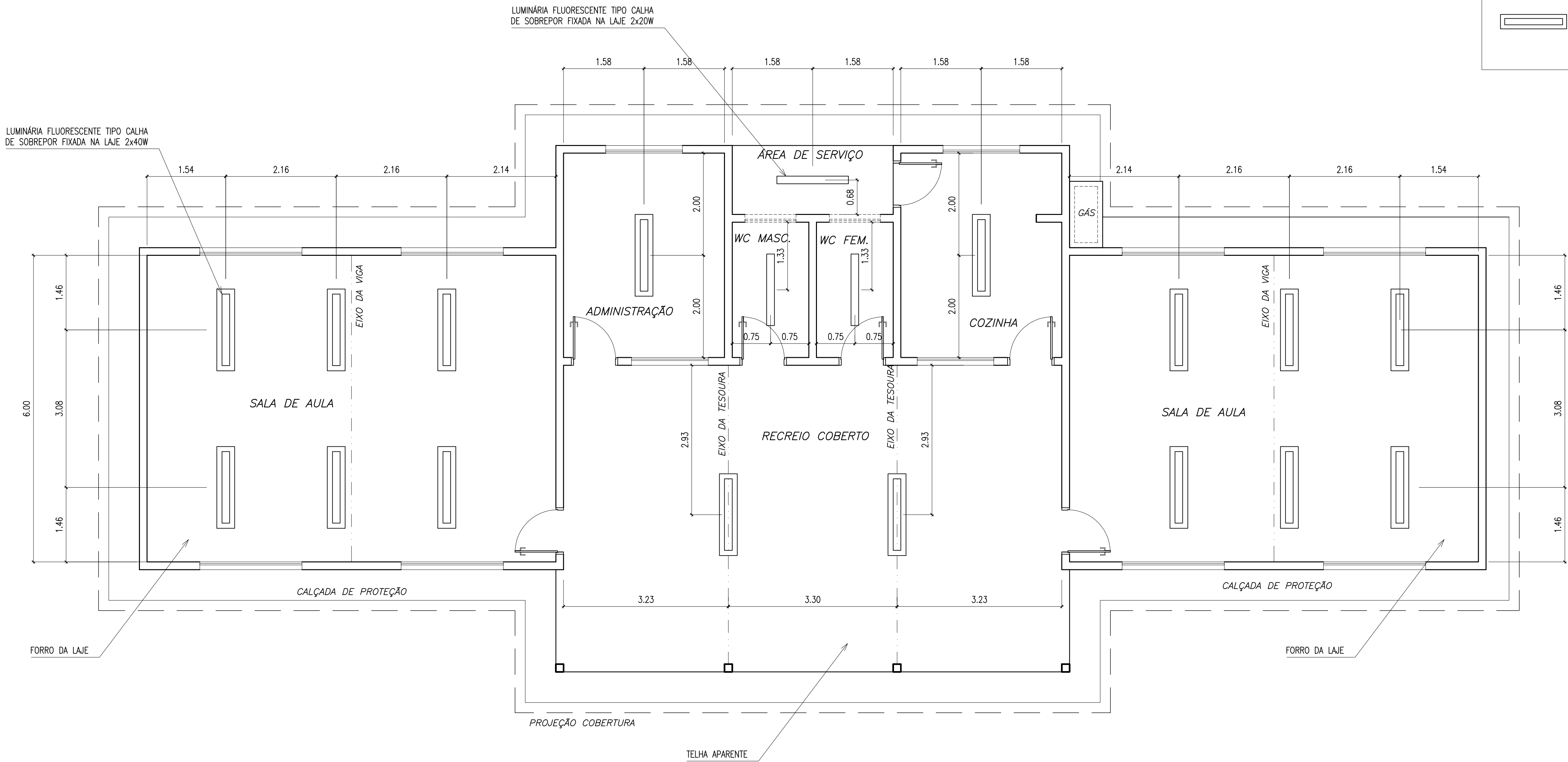
1 PLANTA LUMINOTÉCNICA ESCALA 1/50
