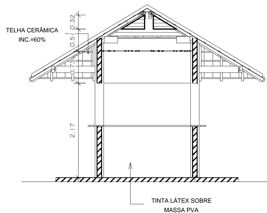
6 CORTE TRANSVERSAL 1 : 50
