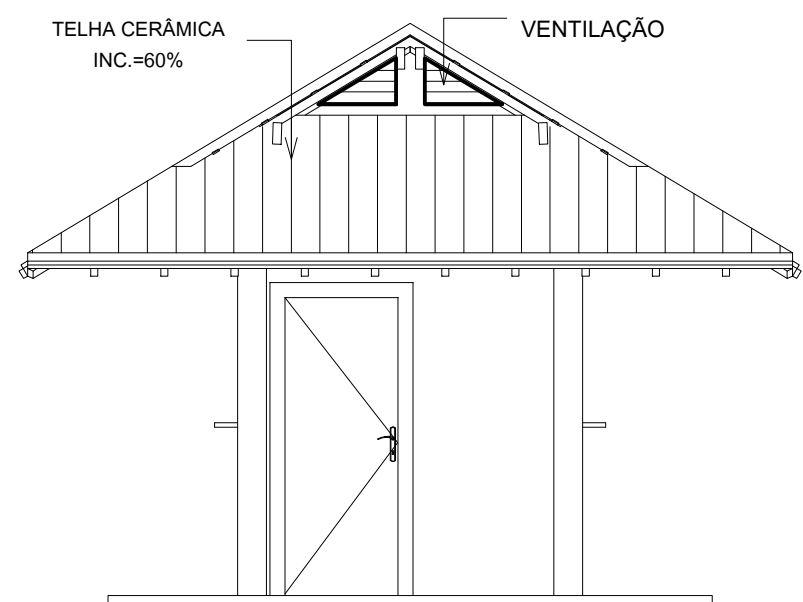
4 FACHADA LATERAL 1 : 50
