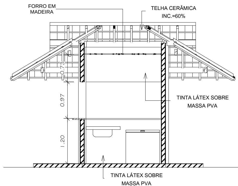
5 CORTE LONGITUDINAL 1 : 50
