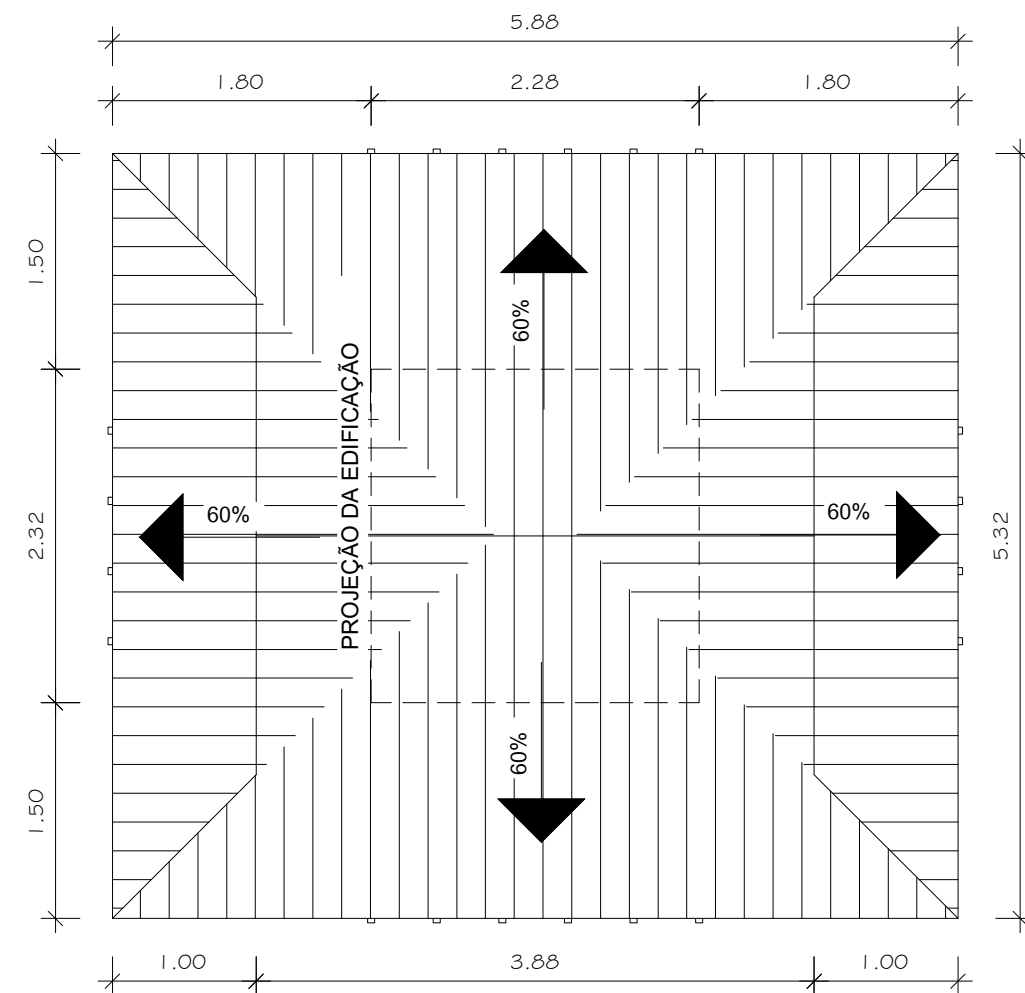
2 03 - COBERTURA 1 : 50
