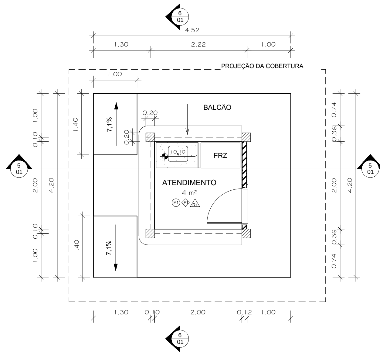
1 02 - TÉRREO 1 : 50
