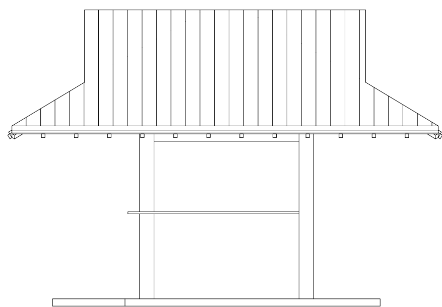
3 FACHADA FRONTAL 1 : 50
