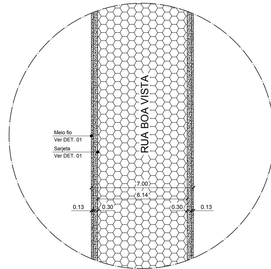
DET. 08 - RUA BOA VISTA S/ ESC.
