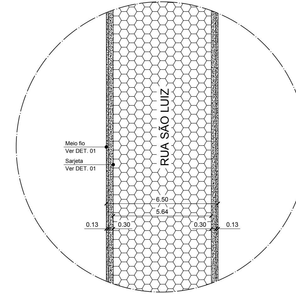
DET. 12 - Travessa São Luiz S/ ESC.
