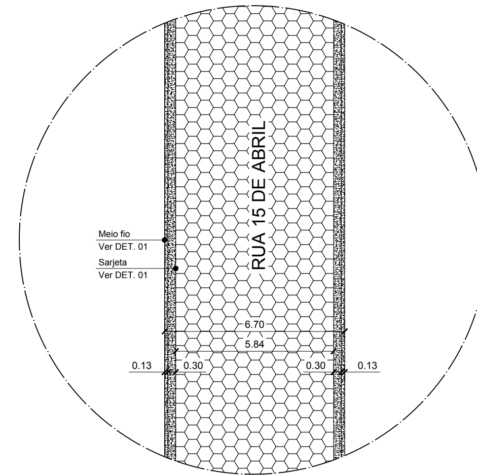
DET. 11 - RUA 15 DE ABRIL (Trecho: Rua Brasília - Rua Alagoas) S/ ESC.
