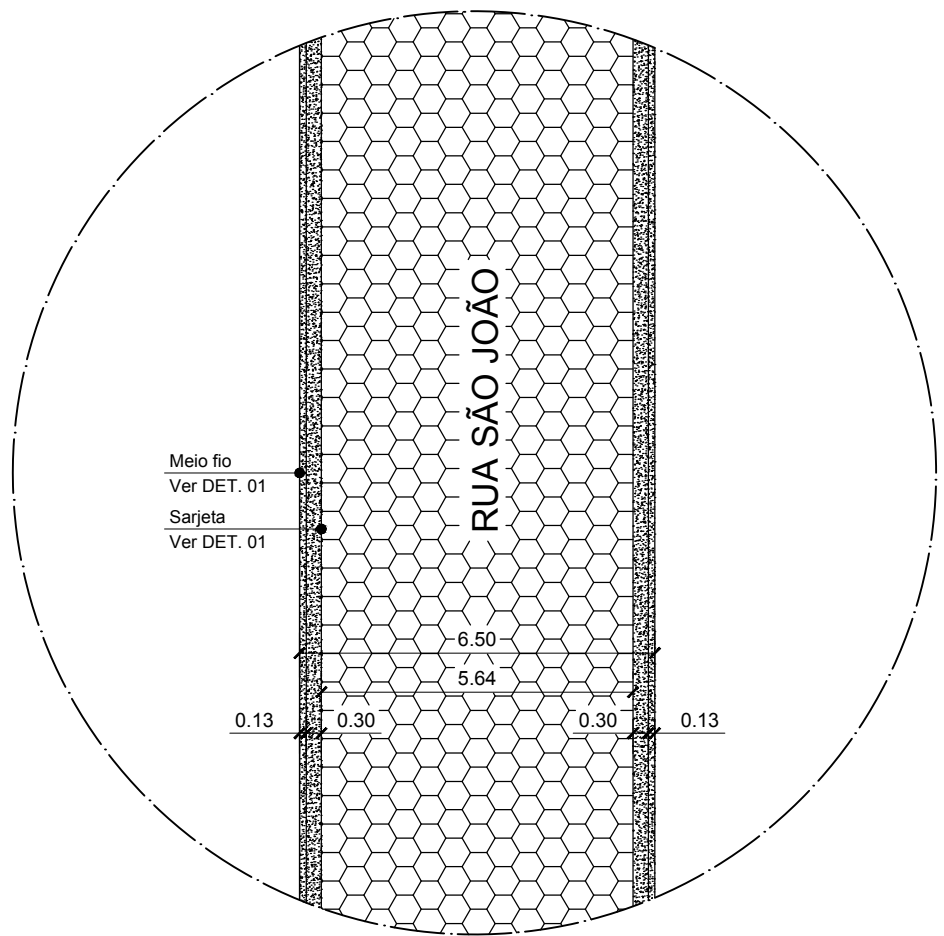
DET. 07 - RUA SÃO JOÃO (Trecho: Rua Paraná - Rua Redenção) S/ ESC.
