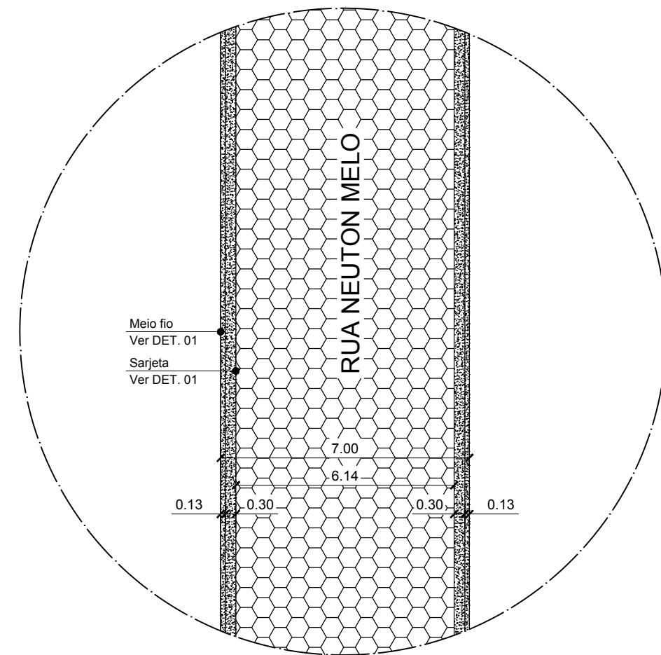
DET. 05 - RUA NEUTON MELO S/ ESC.
