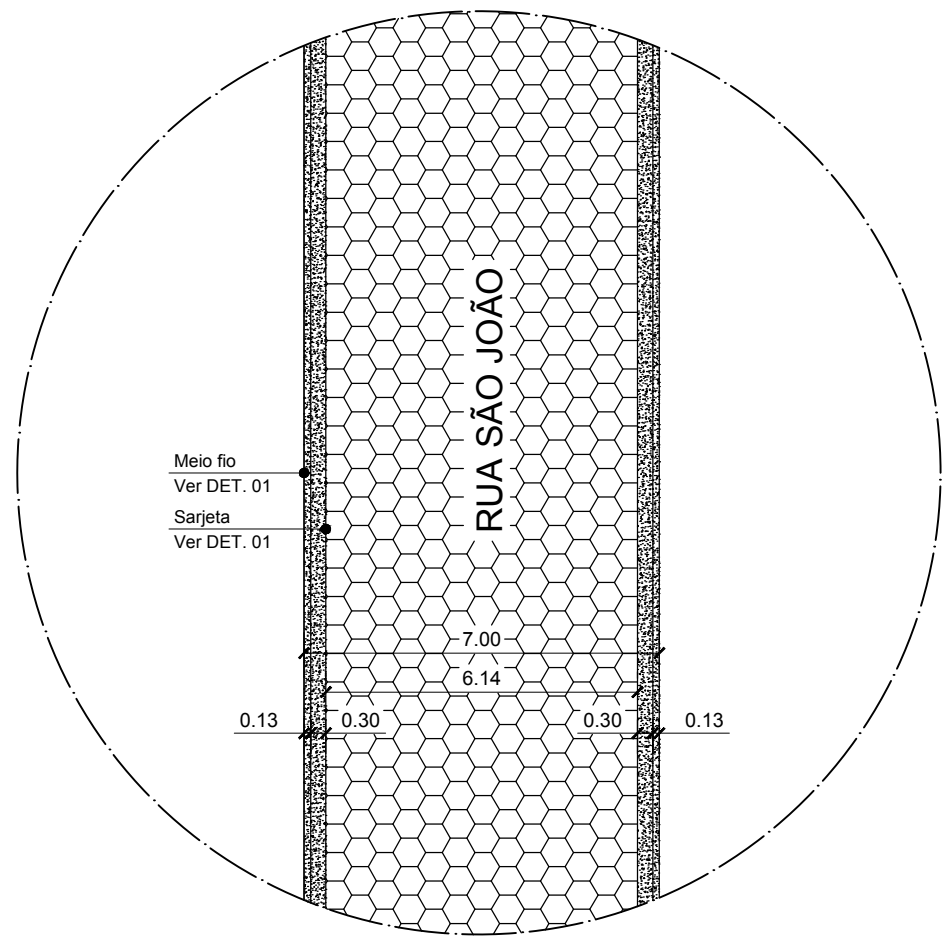
DET. 06 - RUA SÃO JOÃO (Trecho: Rua Bernardino Vieira - Rua Paraná) S/ ESC.
