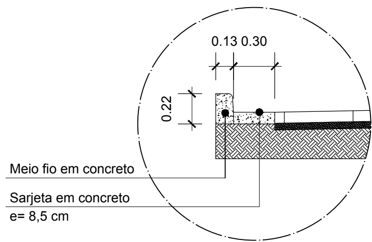
DET. 01 - Meio fio e sarjeta S/ ESC.
