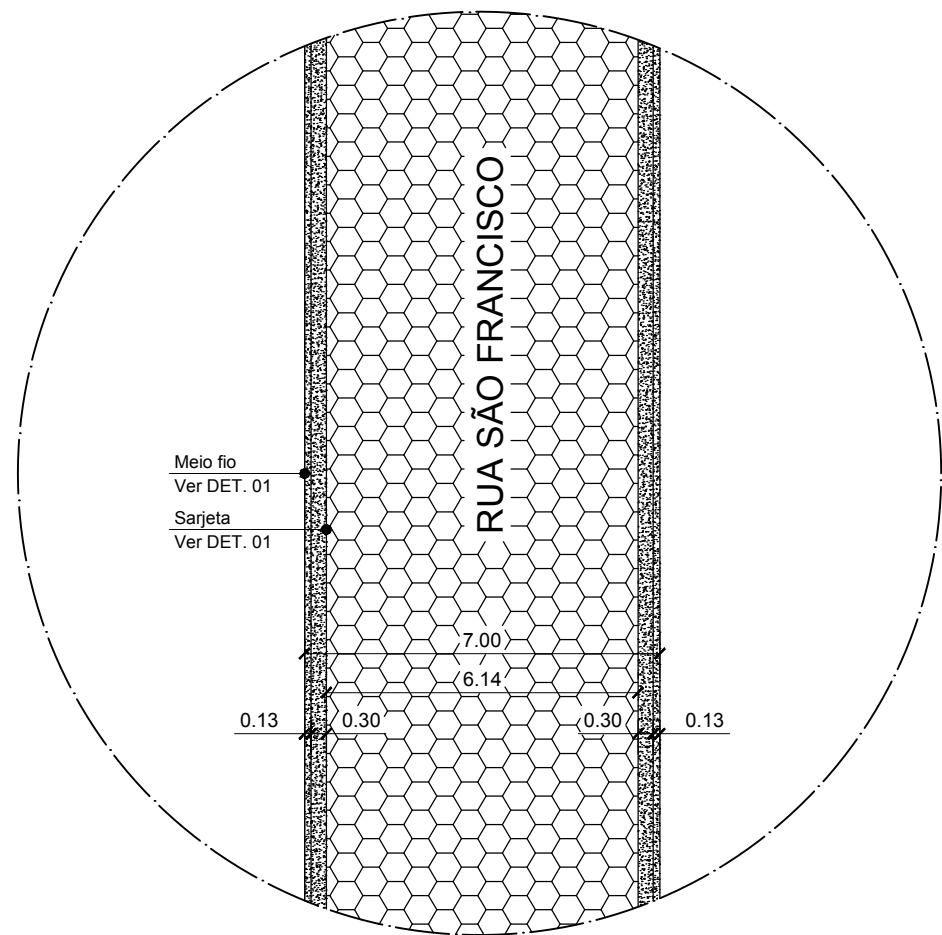
DET. 04 - RUA SÃO FRANCISCO S/ ESC.
