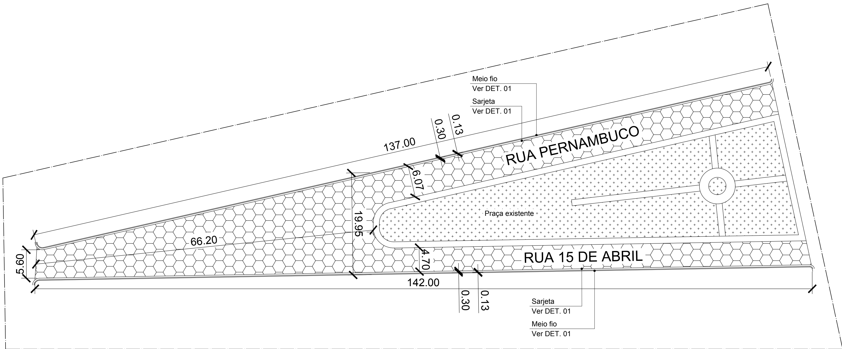
DET. 09 - RUA PERNAMBUCO E RUA 15 DE ABRIL (Trecho: Rua Bernardino Vieira - Rua Brasília) S/ ESC.
