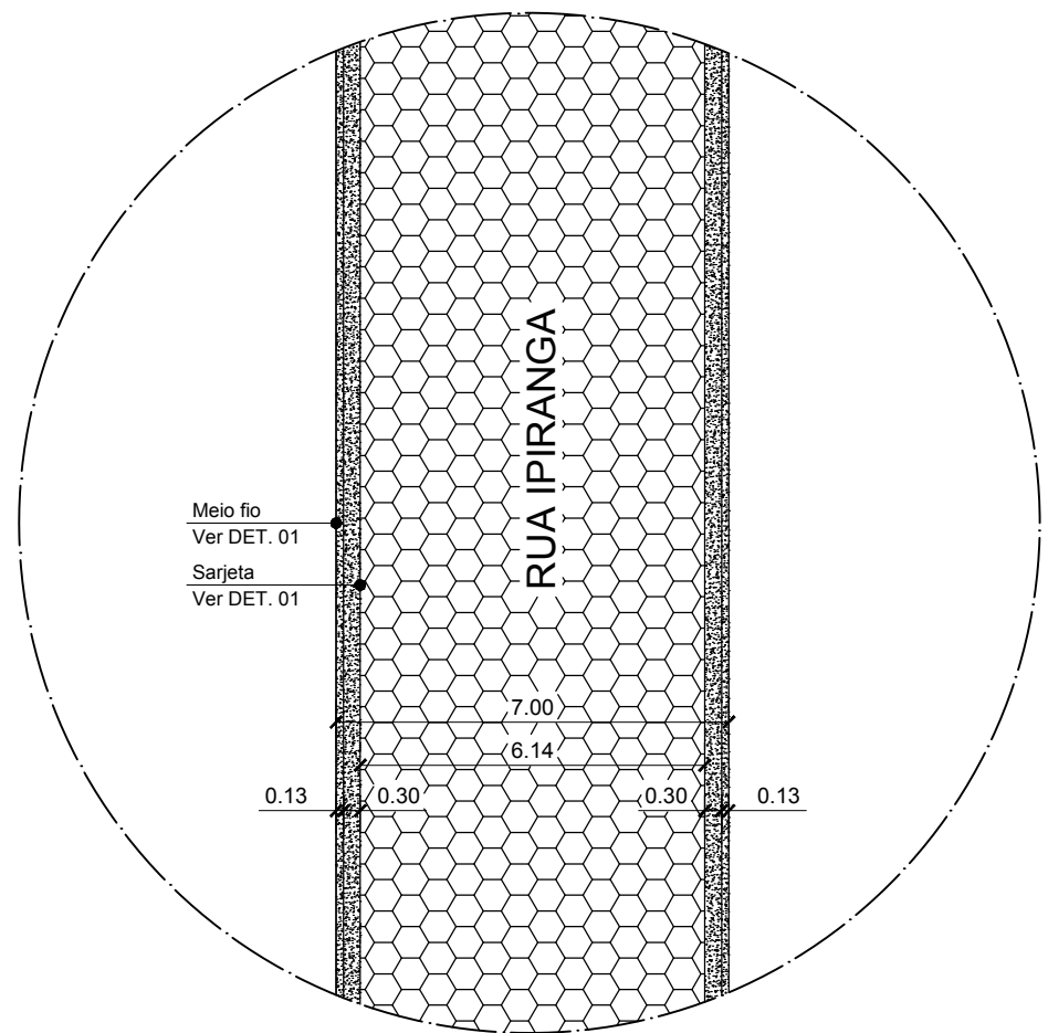
DET. 02 - RUA IPIRANGA S/ ESC.
