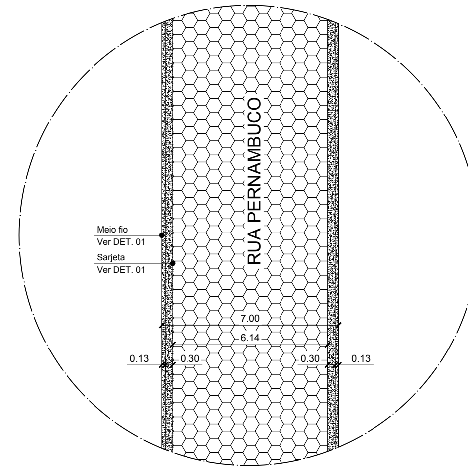
DET. 10 - RUA PERNAMBUCO (Trecho: Rua Brasília - Rua Paraná) S/ ESC.
