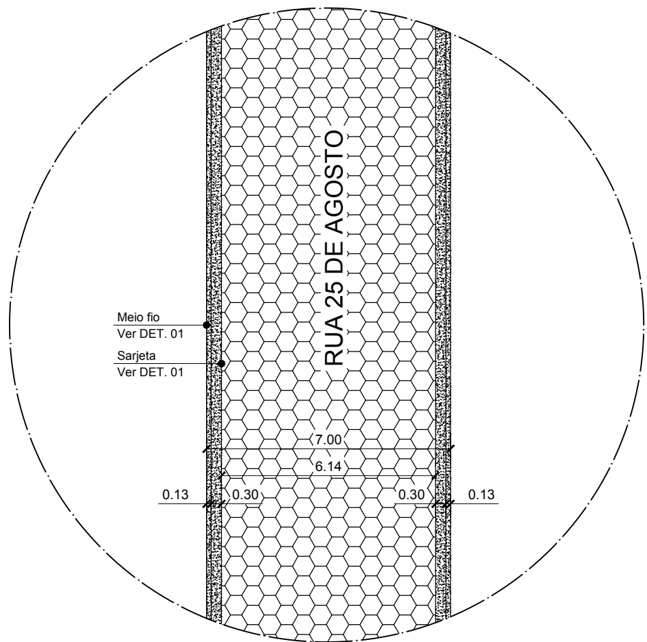
DET. 03 - RUA 25 DE AGOSTO S/ ESC.
