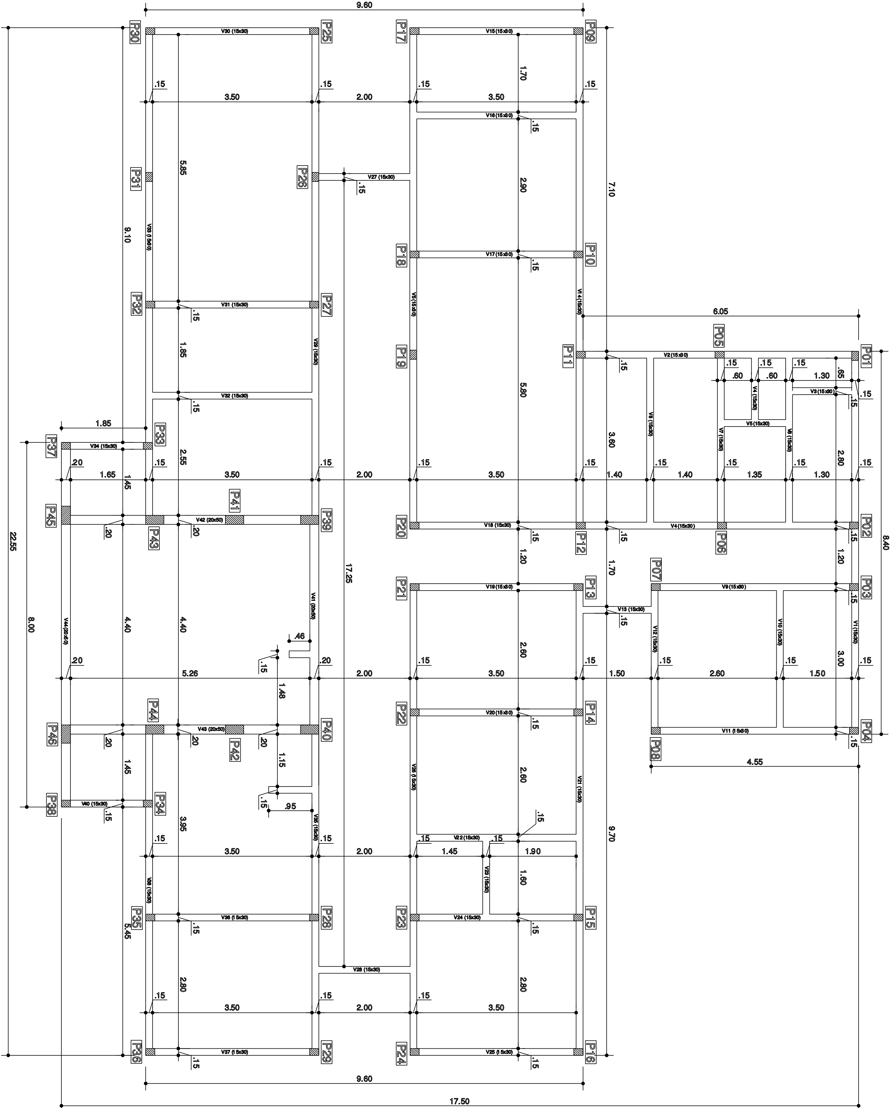
PLANTA DE ARMAÇÃO DE PILARES E CINTAMENTO -
