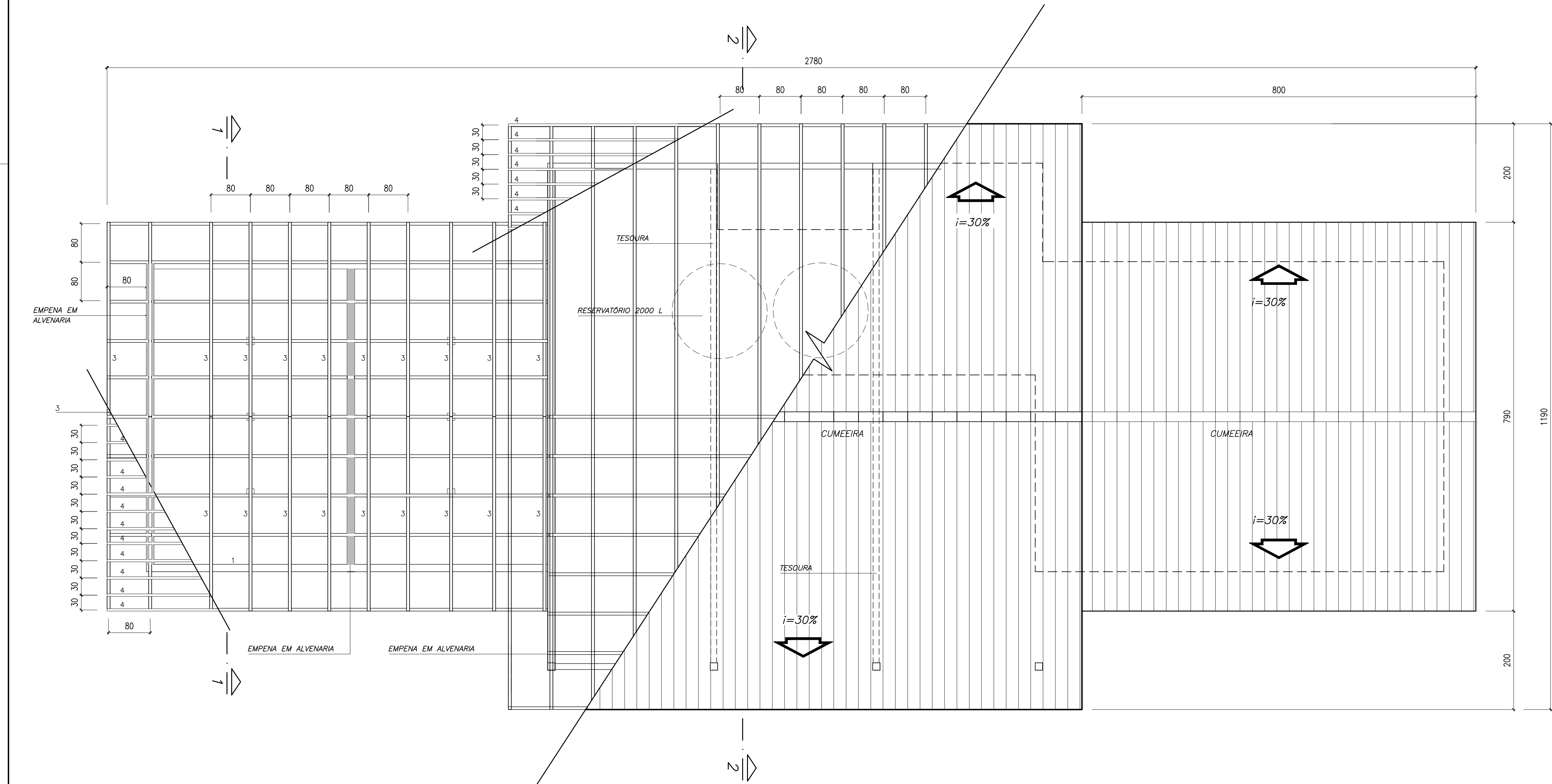
3 PLANTA DE COBERTURA ESCALA 1/50
