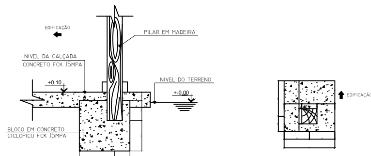
DET. 02 - FUNDAÇÃO/PILAR EM MADEIRA 50x50x50 cm (4x)
