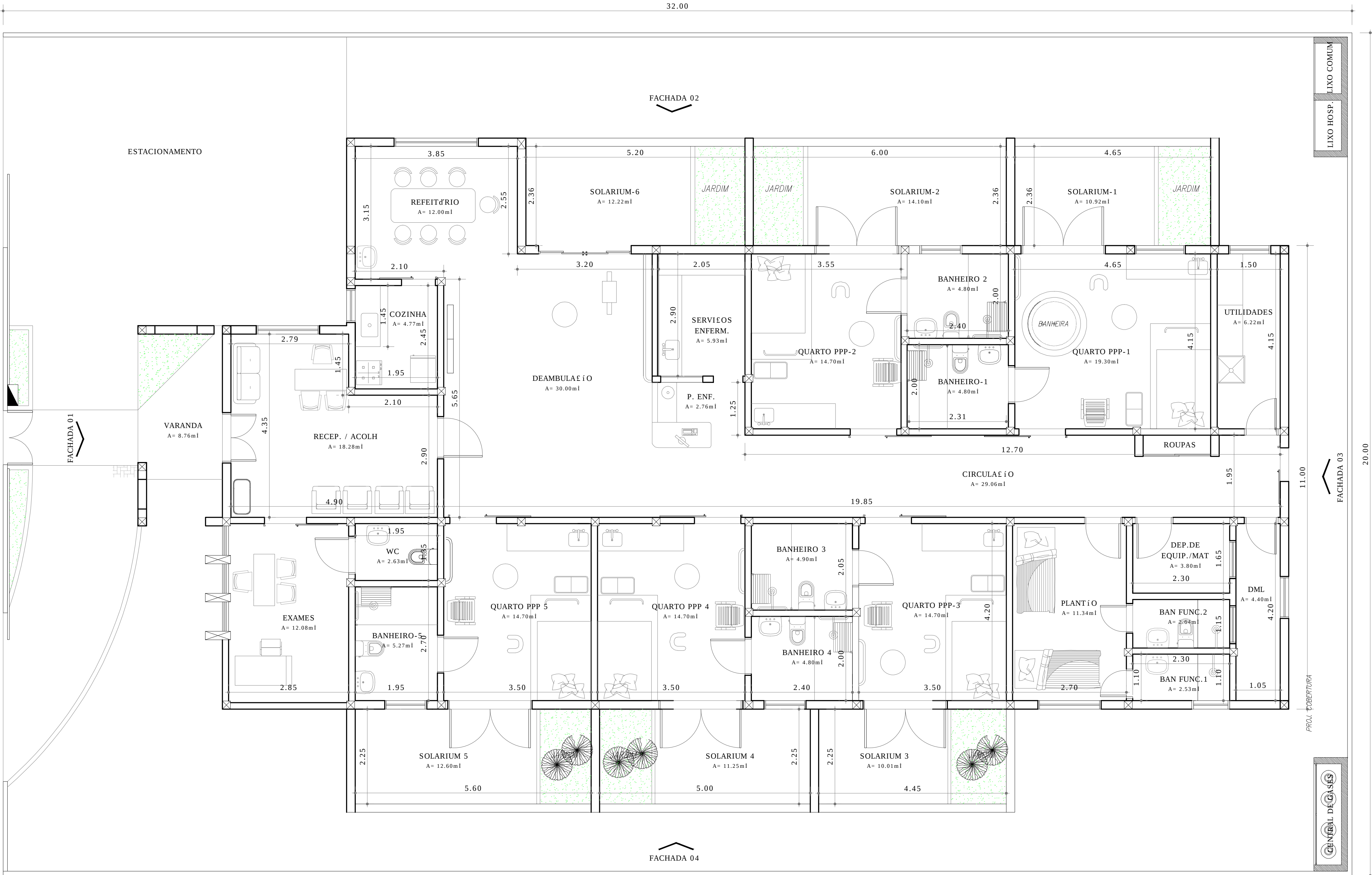
LAYOUT ESC.: 1/50
