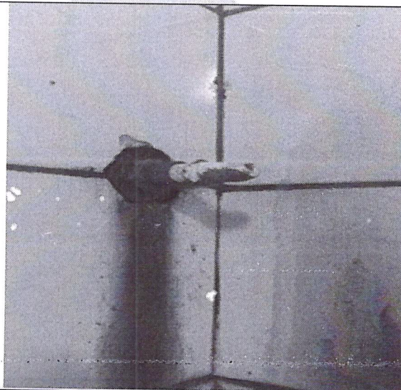
Registros de gaveta danificados e com vazamento.
