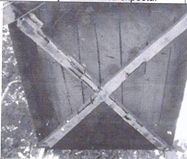
Estrutura da caixa d'água com armadura exposta.
