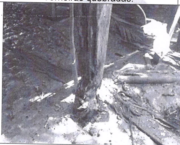
Esteios de sustentação da escola em grave estado de deterioração.
