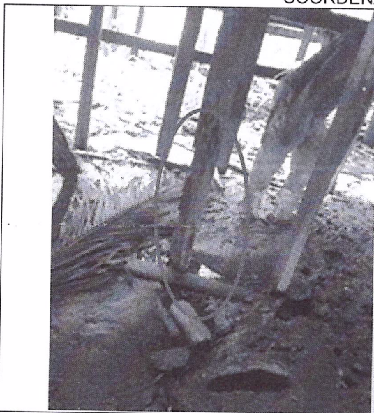
Estrutura de sustentação da escola bastante deteriorada com risco de recalque e desabamento.
