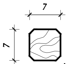
SEÇÃO DO SUPORTE (COTAS EM CENTÍMETROS)
