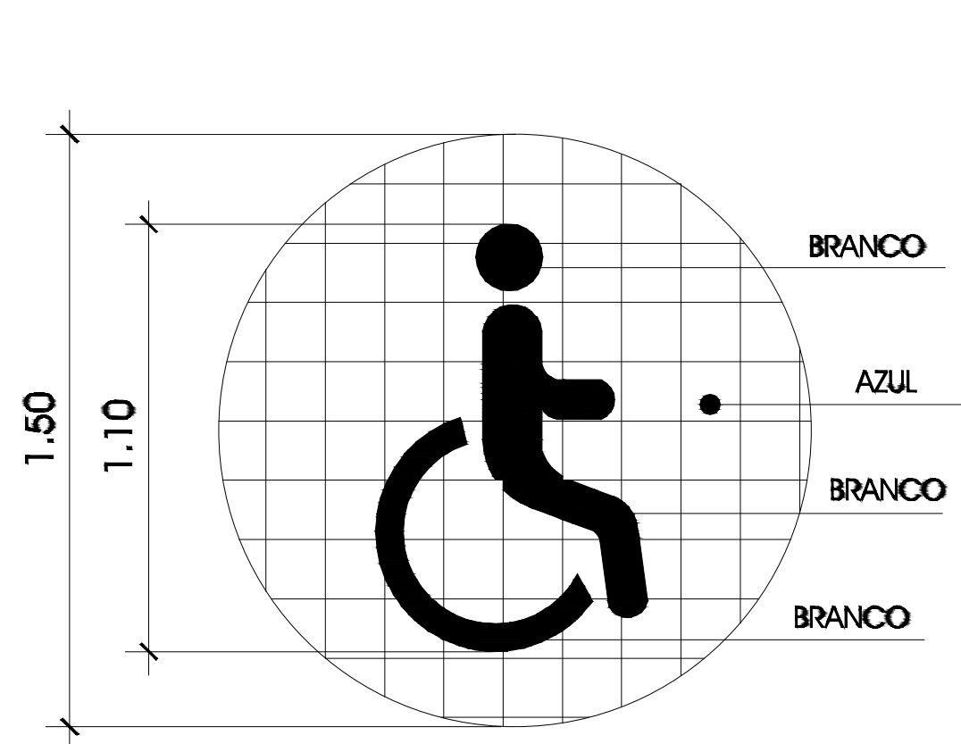
DET. DE PICTOGRAMA / PINTURA - DEFICIENTES FÍSICOS -
