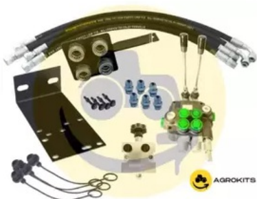
Kit Comando Controle Remoto Duplo Massey Ferguson 275
