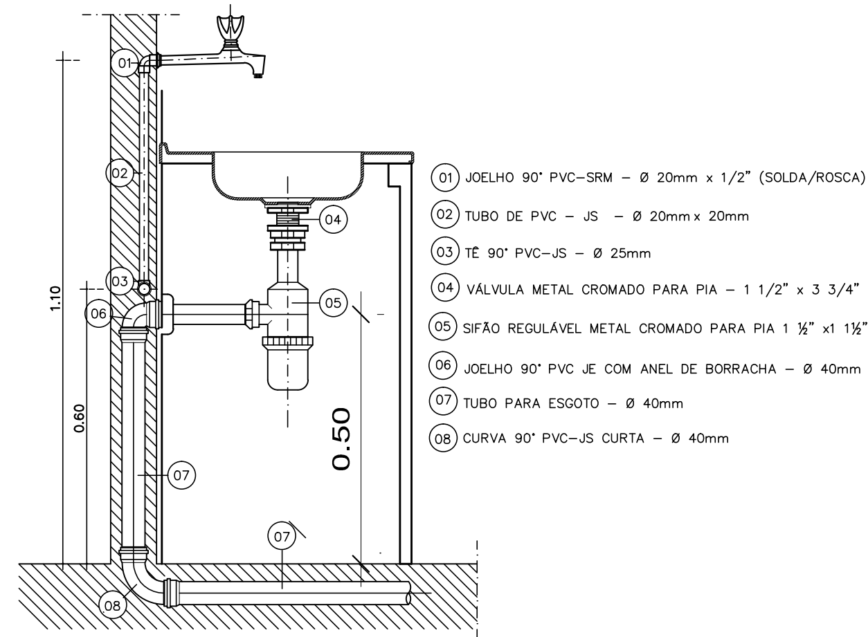
Det. Pia S/Escala
