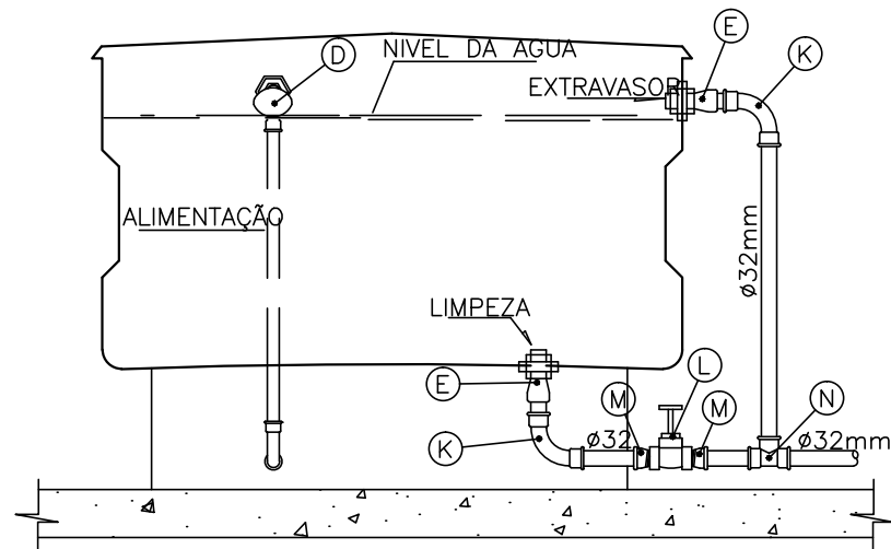
Inst. Caixa D'água S/Escala
