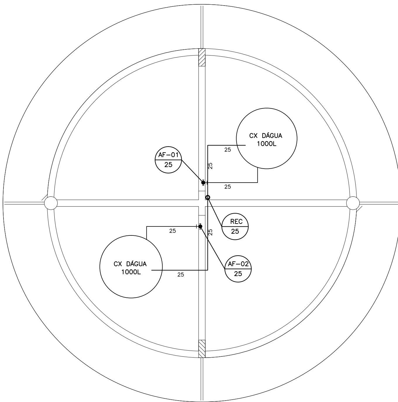
Planta de Distribuição Escala 1/50
