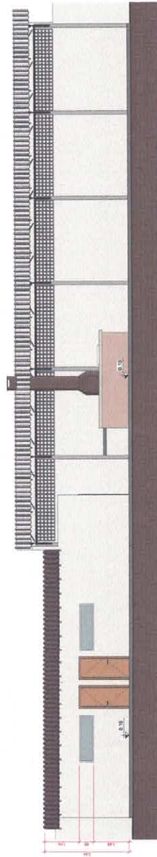
CORTE 2 ESC: 1/75
