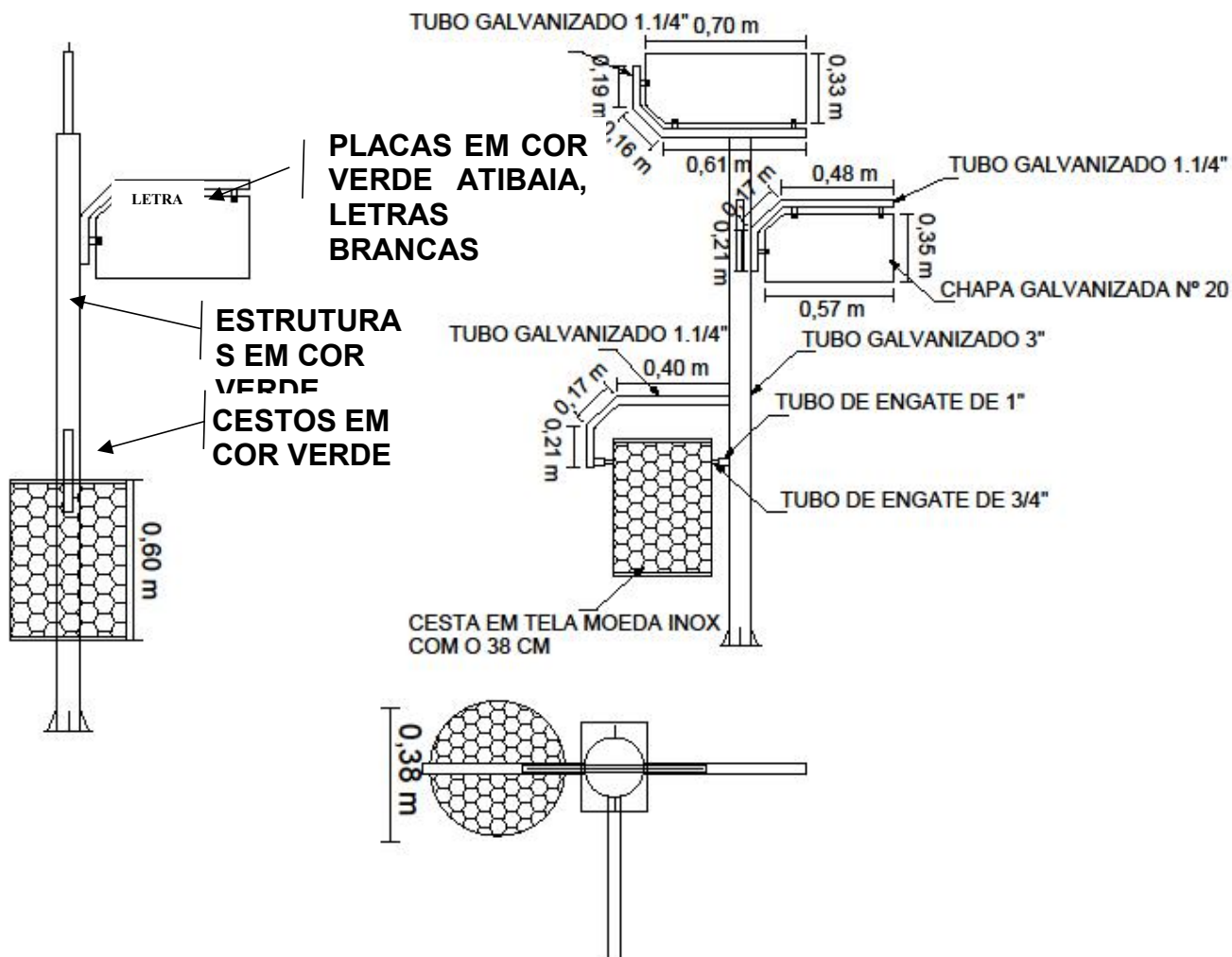
FIG. 04 – POSTE COM UM CESTO REDONDO E DUAS PLACAS
