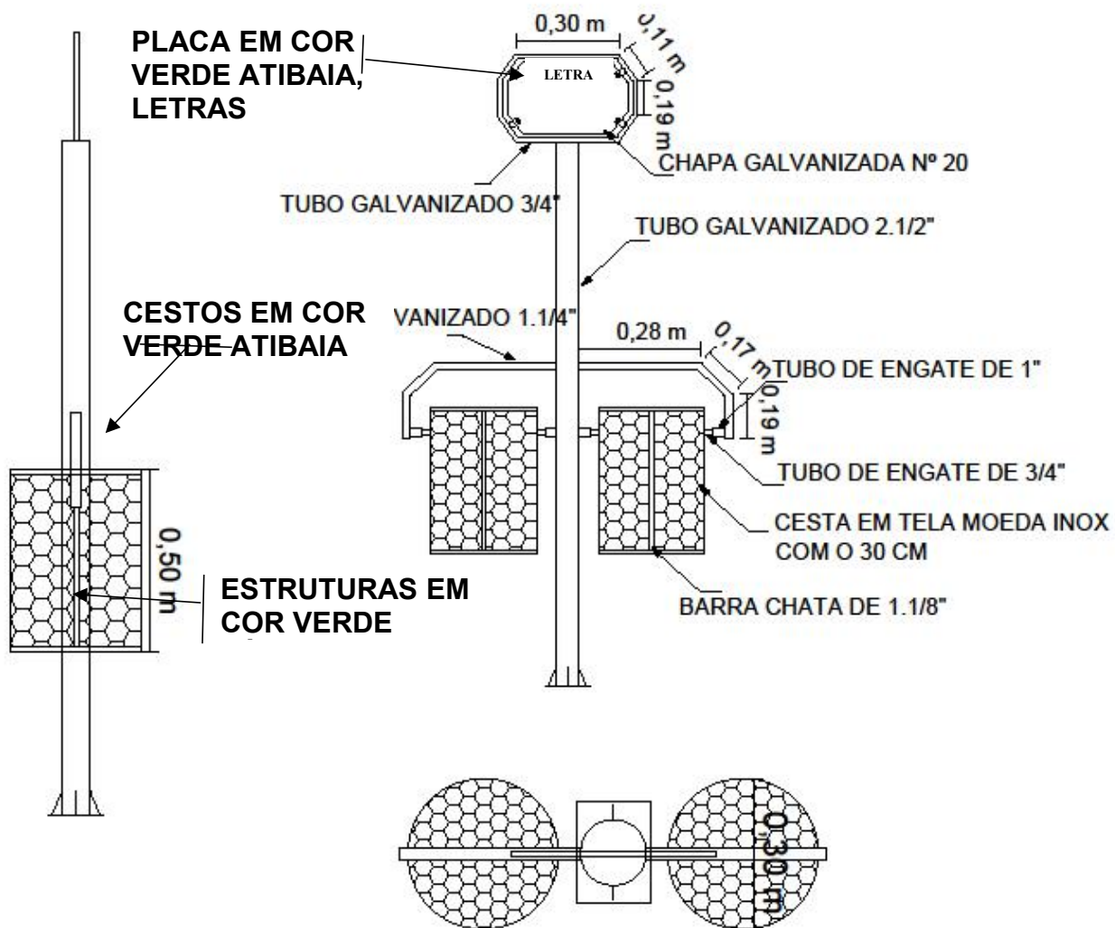
FIG. 03 – POSTE COM DOIS CESTOS REDONDOS E UMA PLACA
