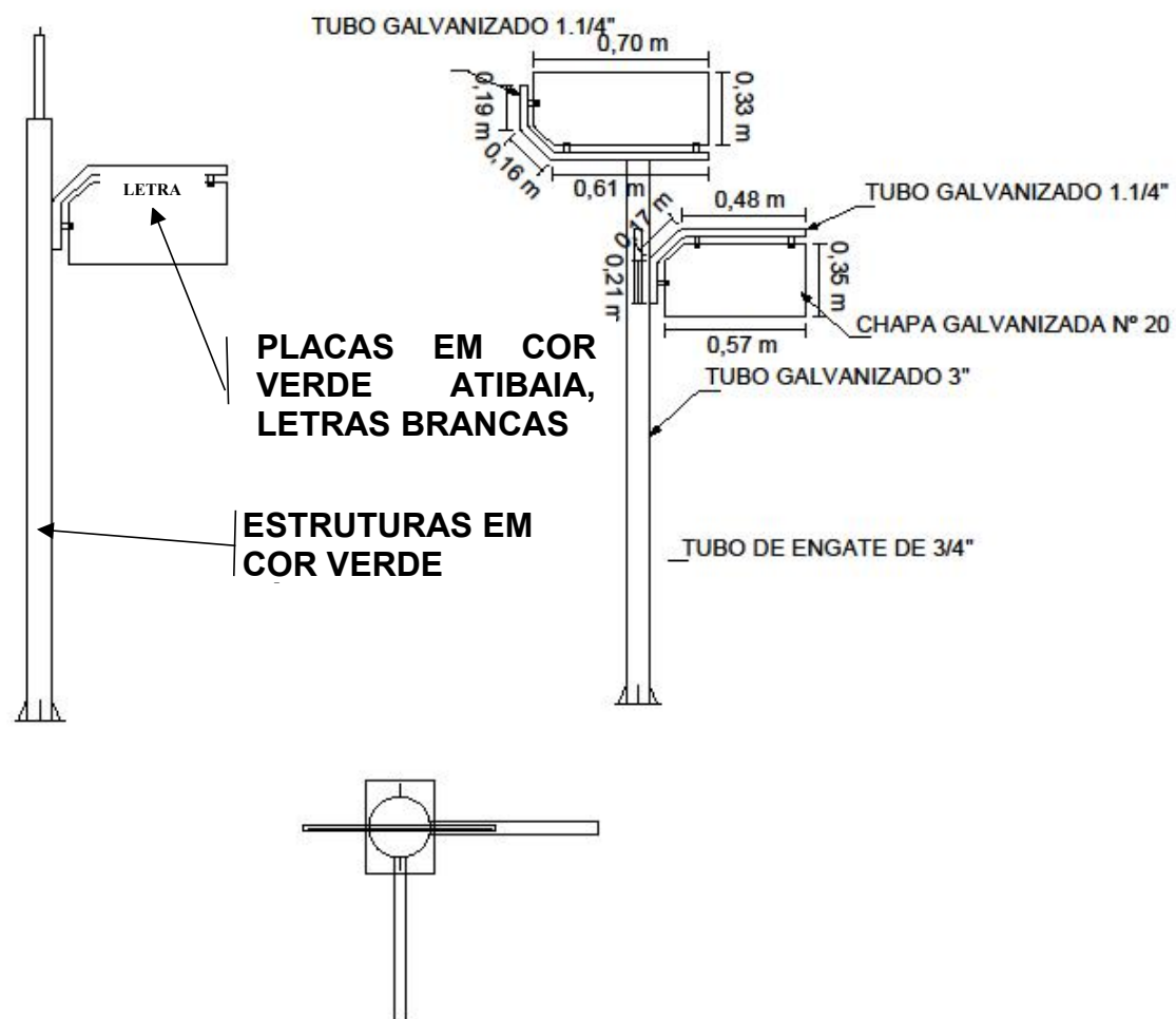
FIG. 05 – POSTE SEM CESTO, COM DUAS PLACAS.
