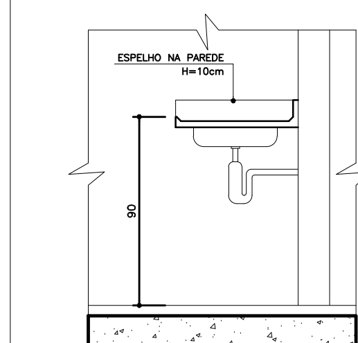
09 Detalhe 1 Esc.: 1:25
