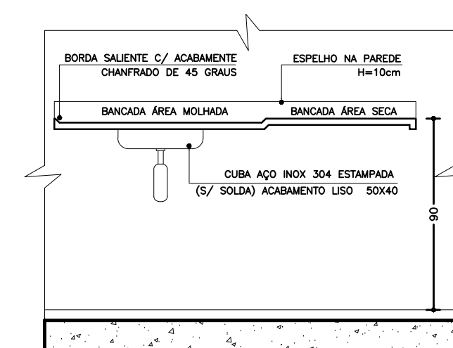
10 Detalhe 2 Esc.: 1:25
