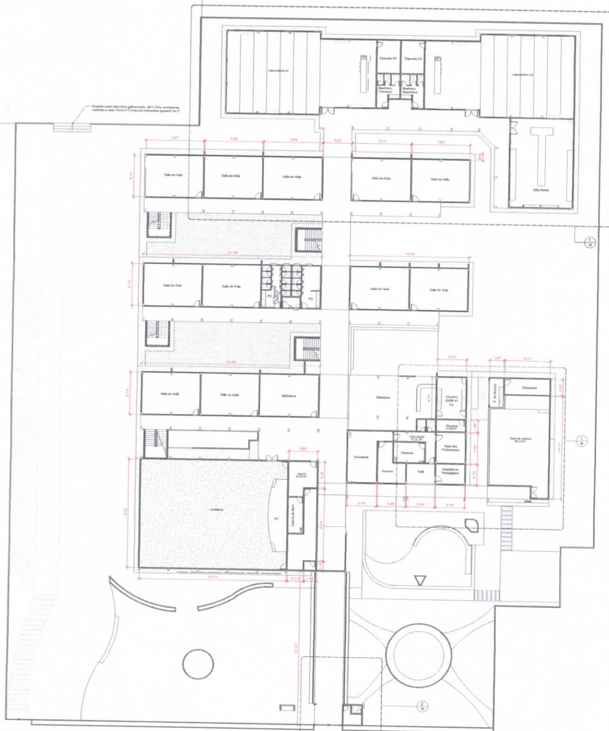
1 PLANTA BAIXA PAV. TERREO
