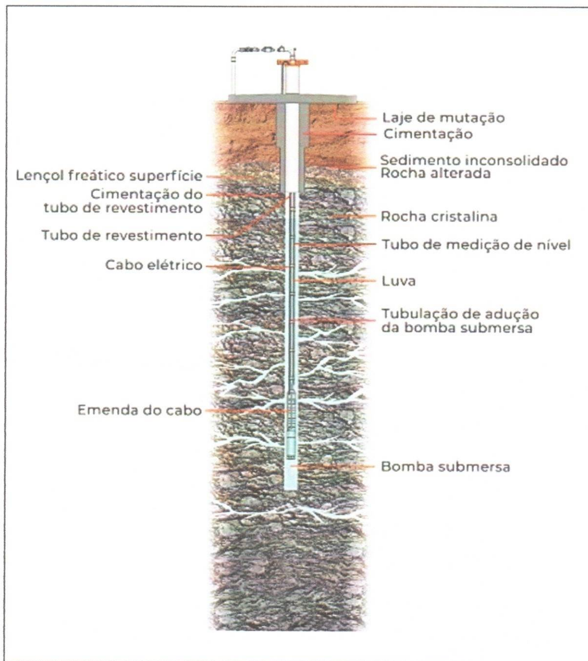
FIGURA 2: PERFIL CONSTRUTIVO DO POÇO.
