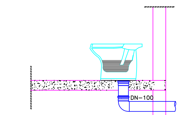
DETALHE DA INSTALAÇÃO DO VASO
