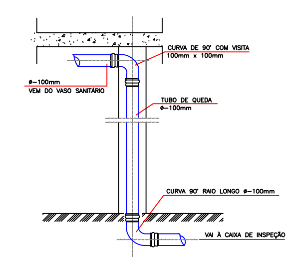
DETALHE-04 TUBO DE QUEDA
