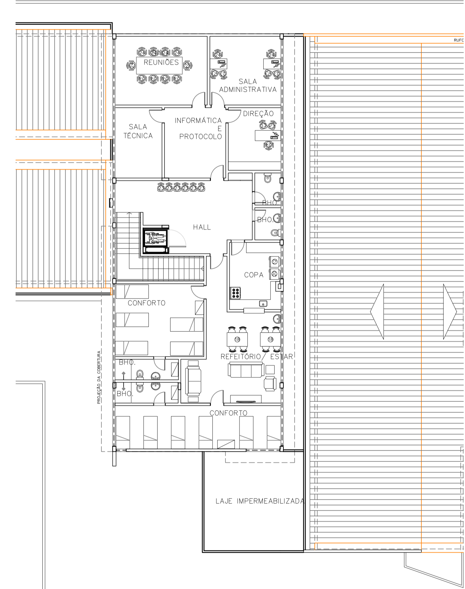
LAYOUT - PAV. SUPERIOR ESC.: 1/100
