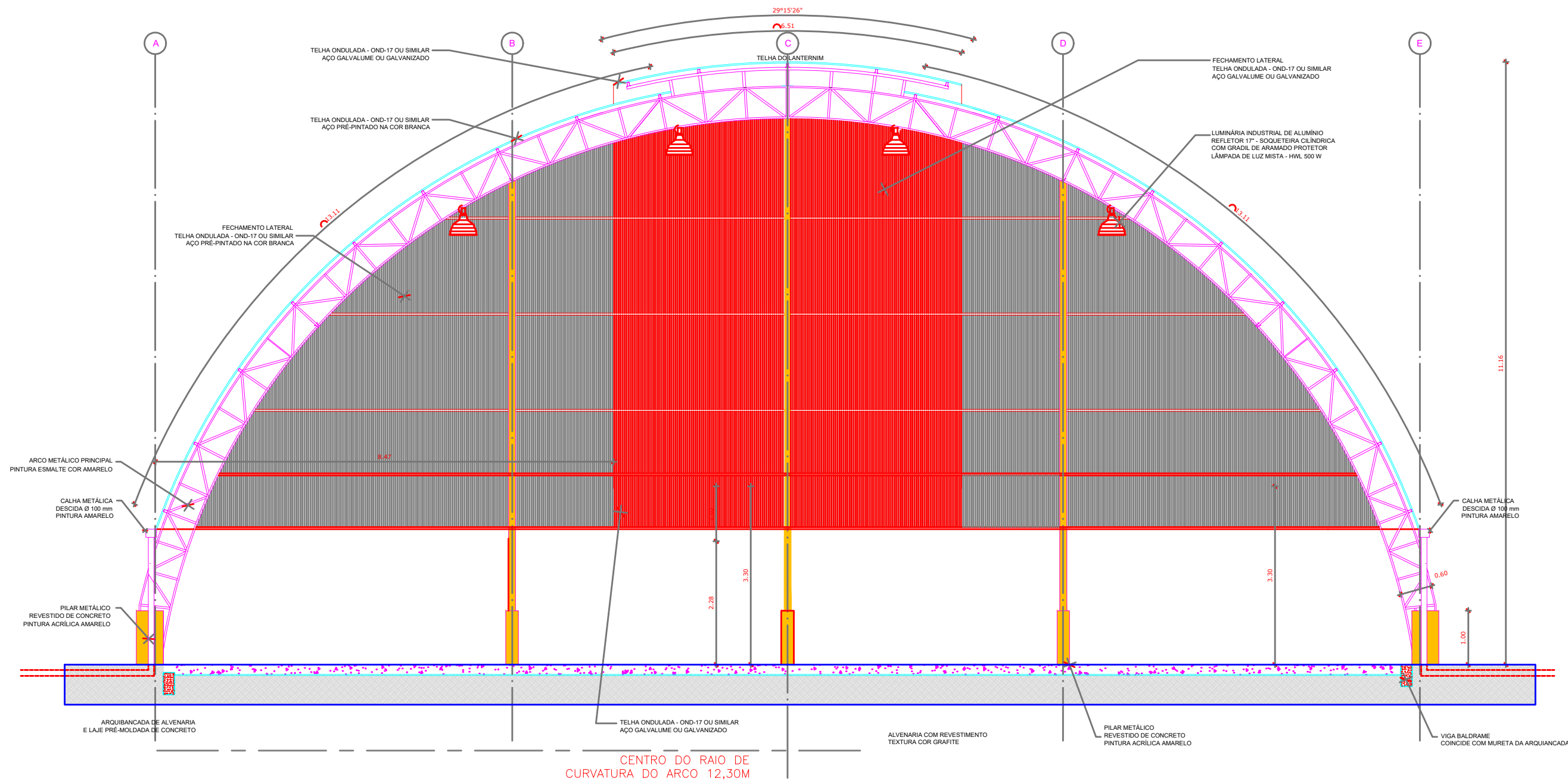
CORTE B/B ESCALA 1:125
