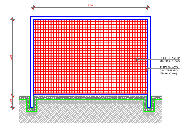
BALISA FUTEBOL VISTA FRONTAL ESCALA 1:25
