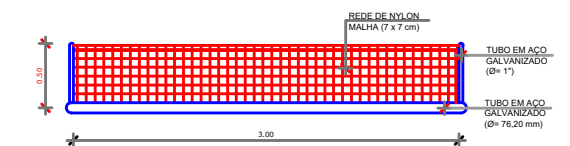
BALISA FUTEBOL PLANTA ESCALA 1:25
