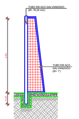
BALISA FUTEBOL VISTA LATERAL ESCALA 1:25
