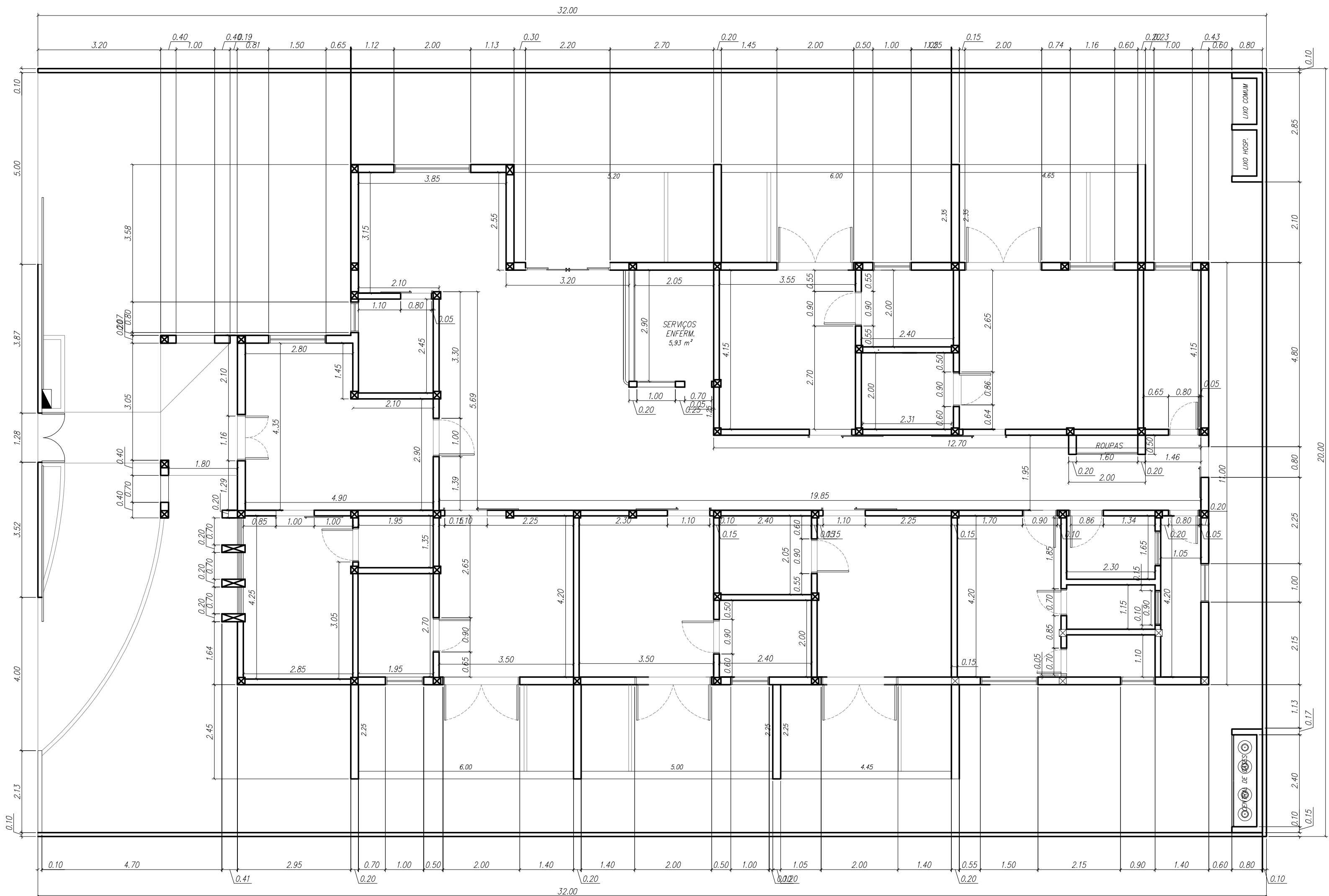
COTAS Esc. 1:75
