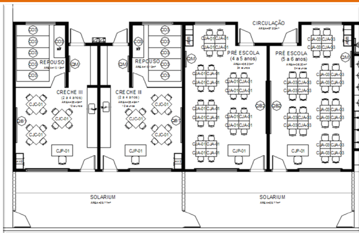
Planta Baixa - Layout
