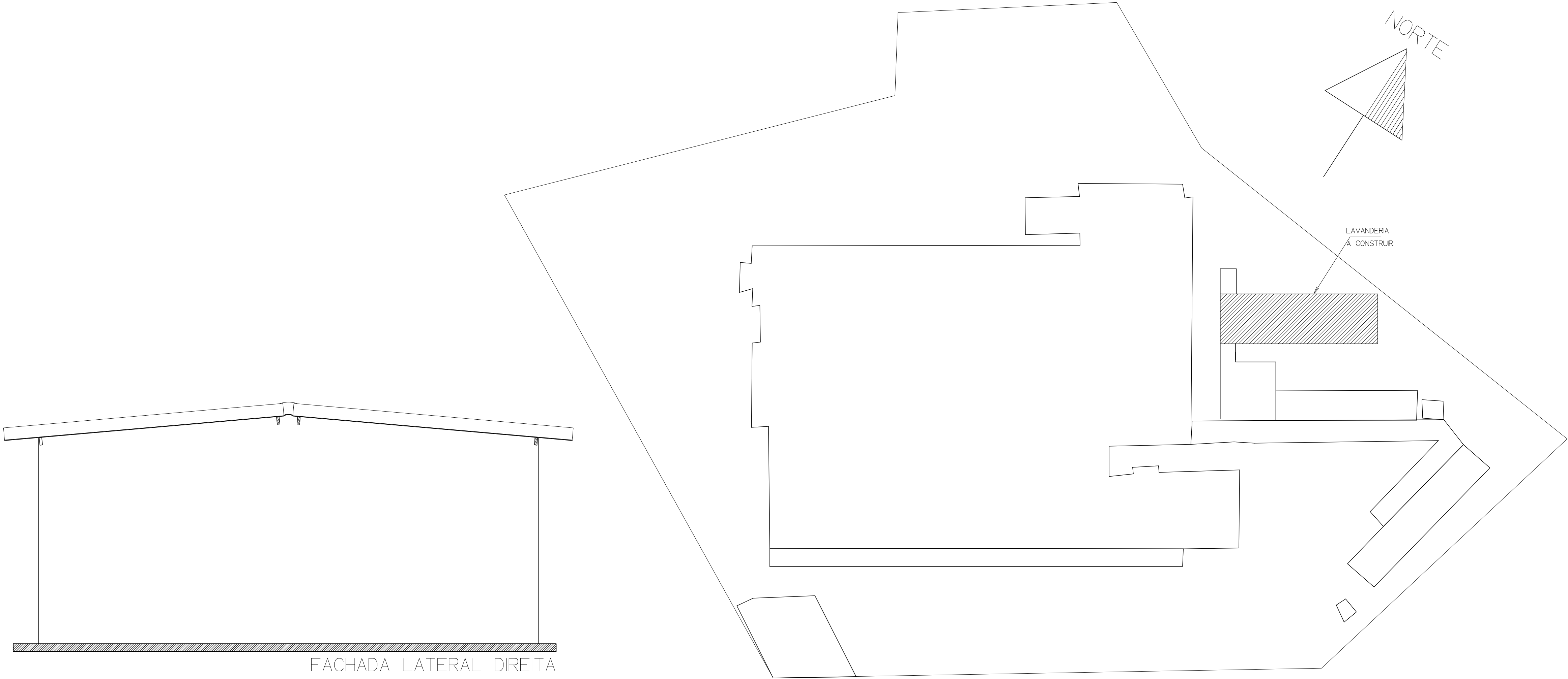
PLANTA DE LOCAÇÃO ESCALA – 1:500
