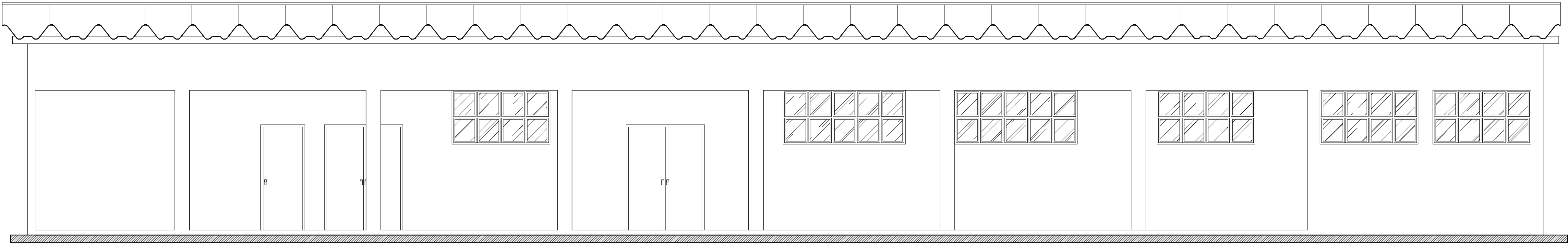
FACHADA FRONTAL ESCALA – 1:50
