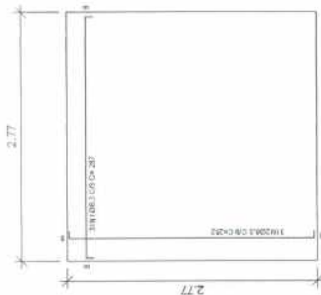
ARMADURA NEGATIVA
