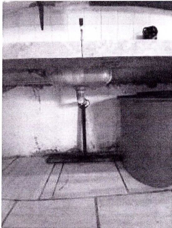
Figura 13 – bancada de concreto revestida da Copa/ cozinha, Tubulação Sustentada de forma inadequada.
