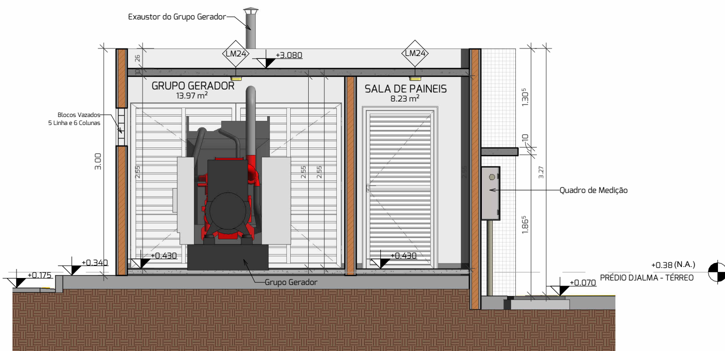
6 SUBESTAÇÃO - SEÇÃO B ESCALA 1: 50
