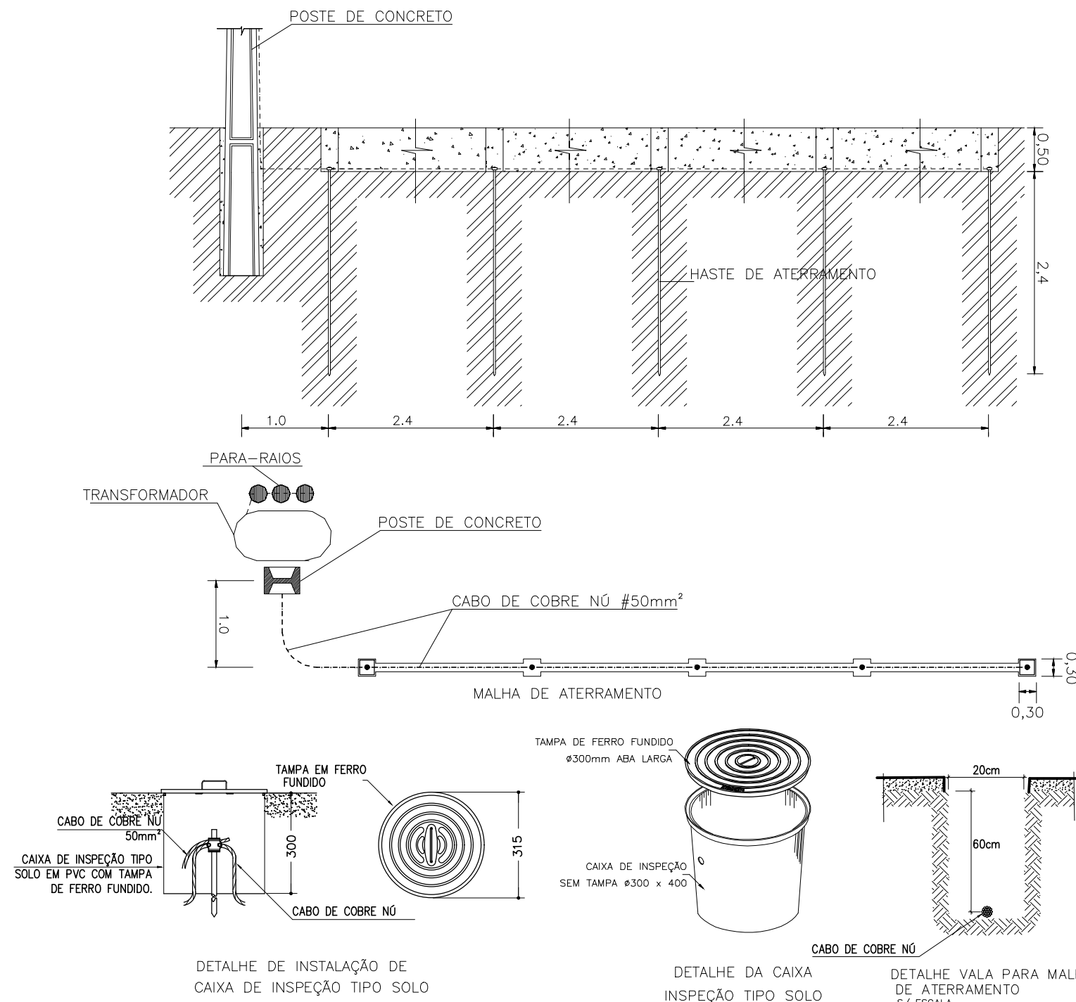
DETALHE-MALHA DE ATERRAMENTO S/ESC.
