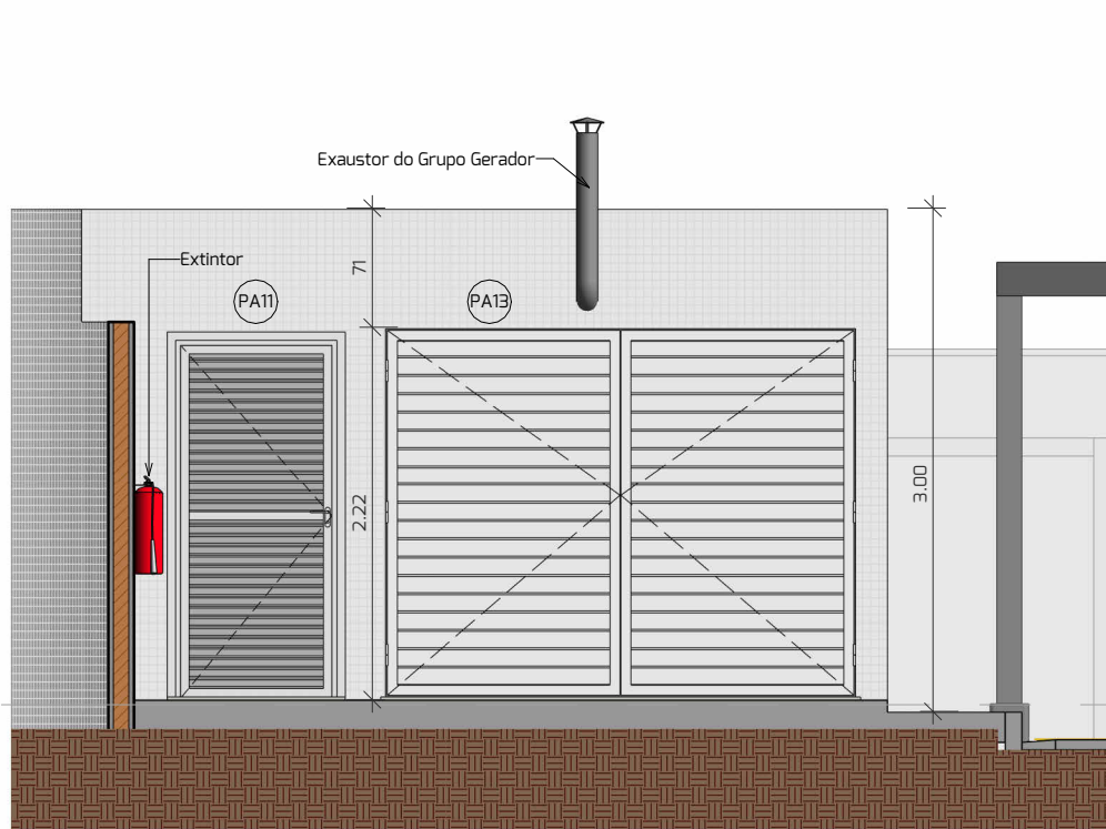
2 SUBESTAÇÃO - FACHADA B ESCALA 1: 50
