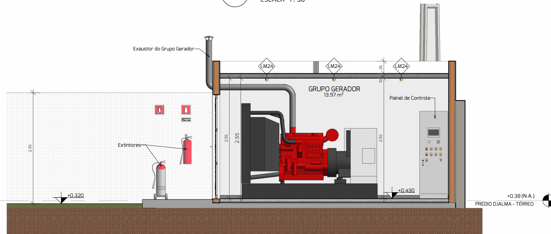
5 SUBESTAÇÃO - SEÇÃO A ESCALA 1: 50
