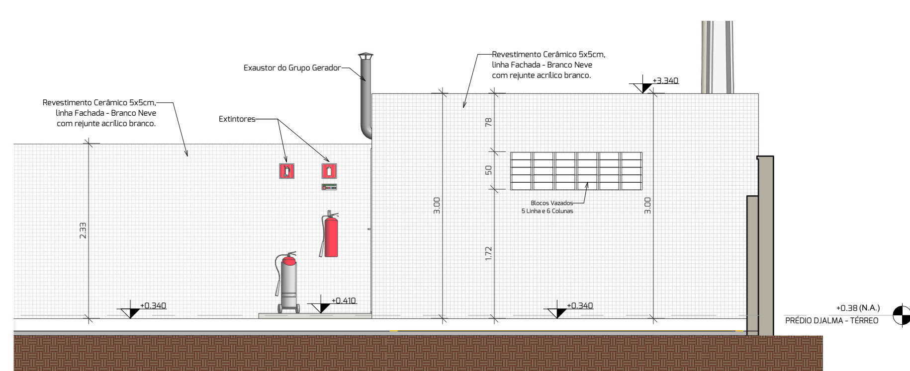
3 SUBESTAÇÃO - FACHADA C ESCALA 1: 50
